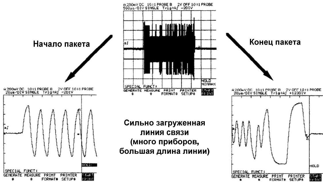
Рисунок 33 Типичная осциллограмма сигнала при большой нагрузке линии связи
