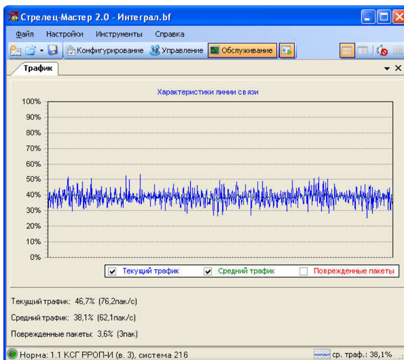
Рисунок 23 Внешний вид ПО в режиме "Обслуживание"
