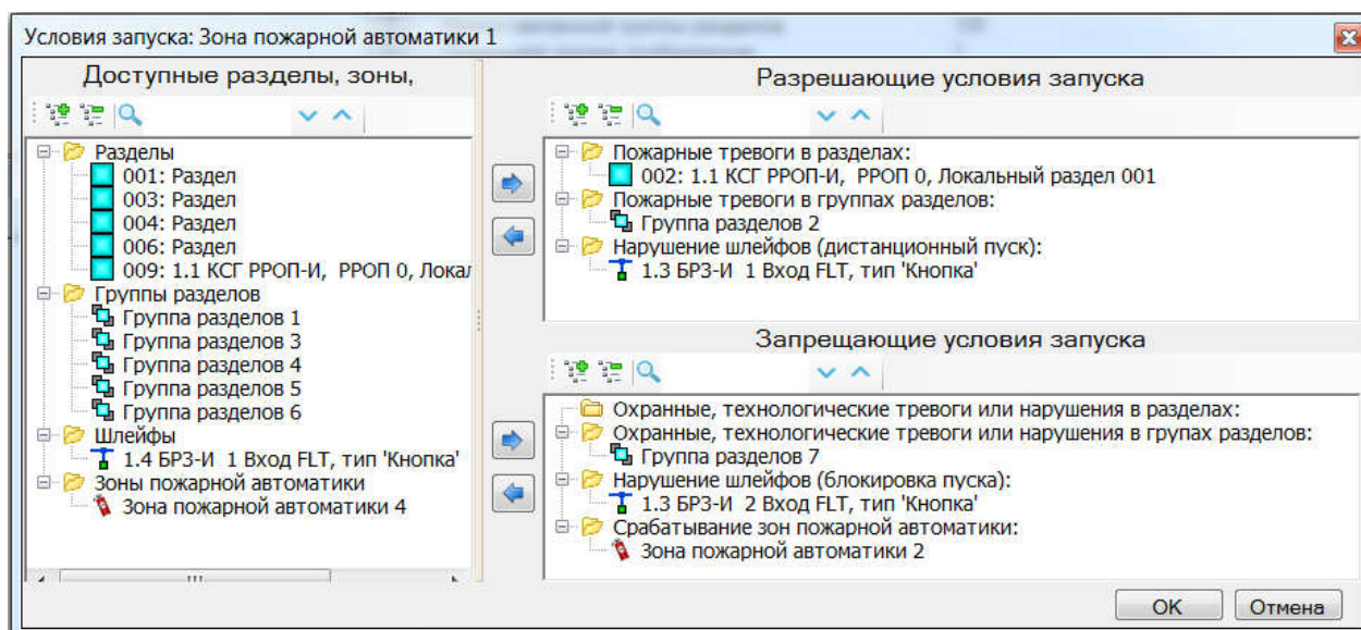
Рисунок 19 Пример формирования условий запуска зоны пожарной автоматики
