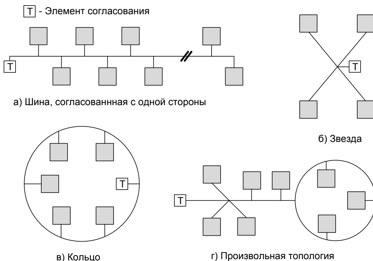
Рисунок 3 Реализуемые сетевые топологии в ТР/FT-10
