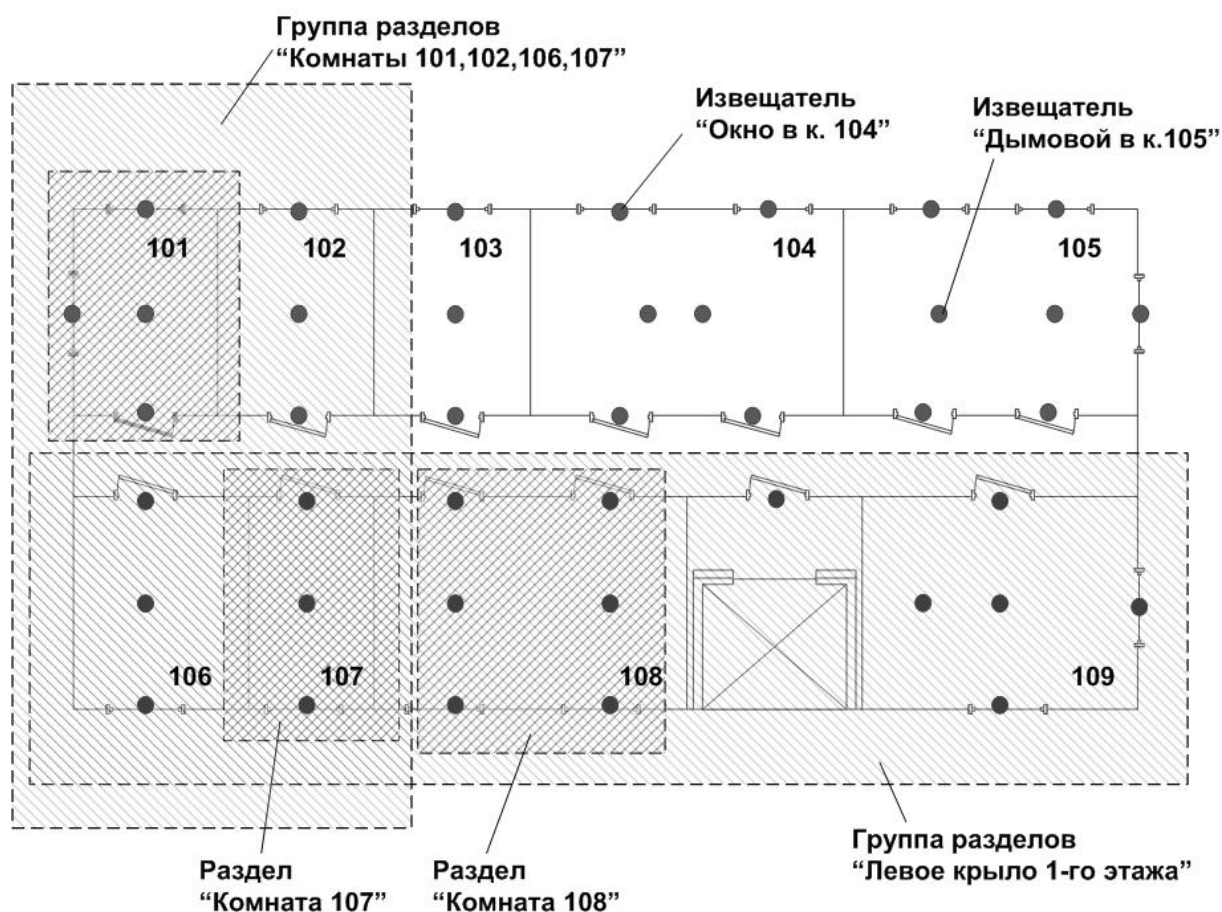
Рисунок 14 Пример организации разделов и групп разделов
