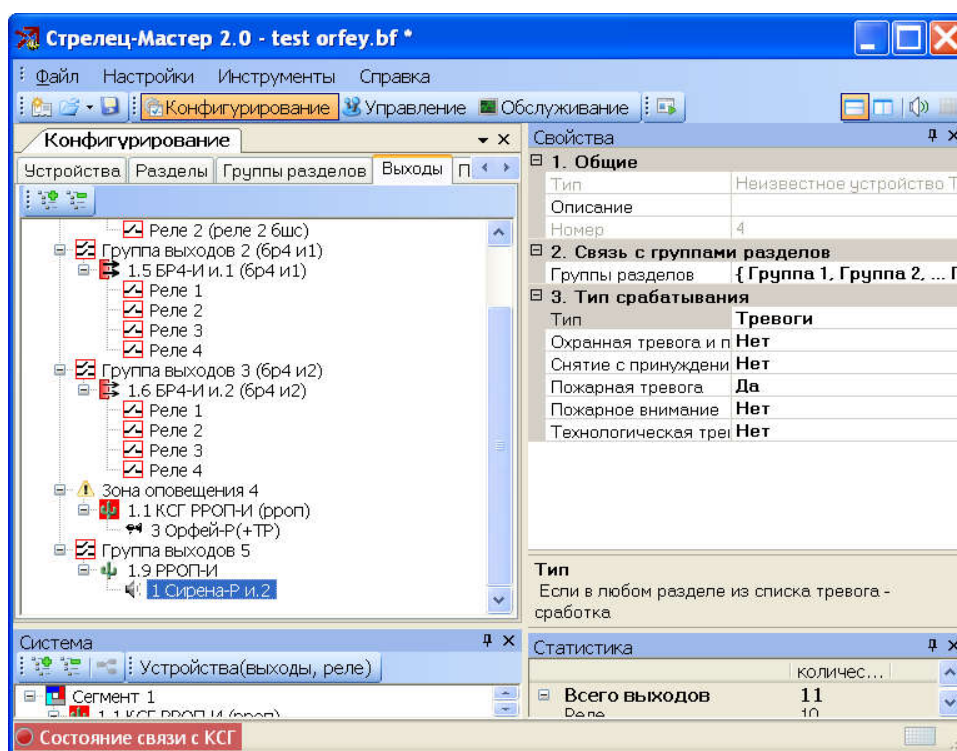
Рисунок 17 Настройка "Сирены-Р" для срабатывания по условиям сегмента ИСБ
