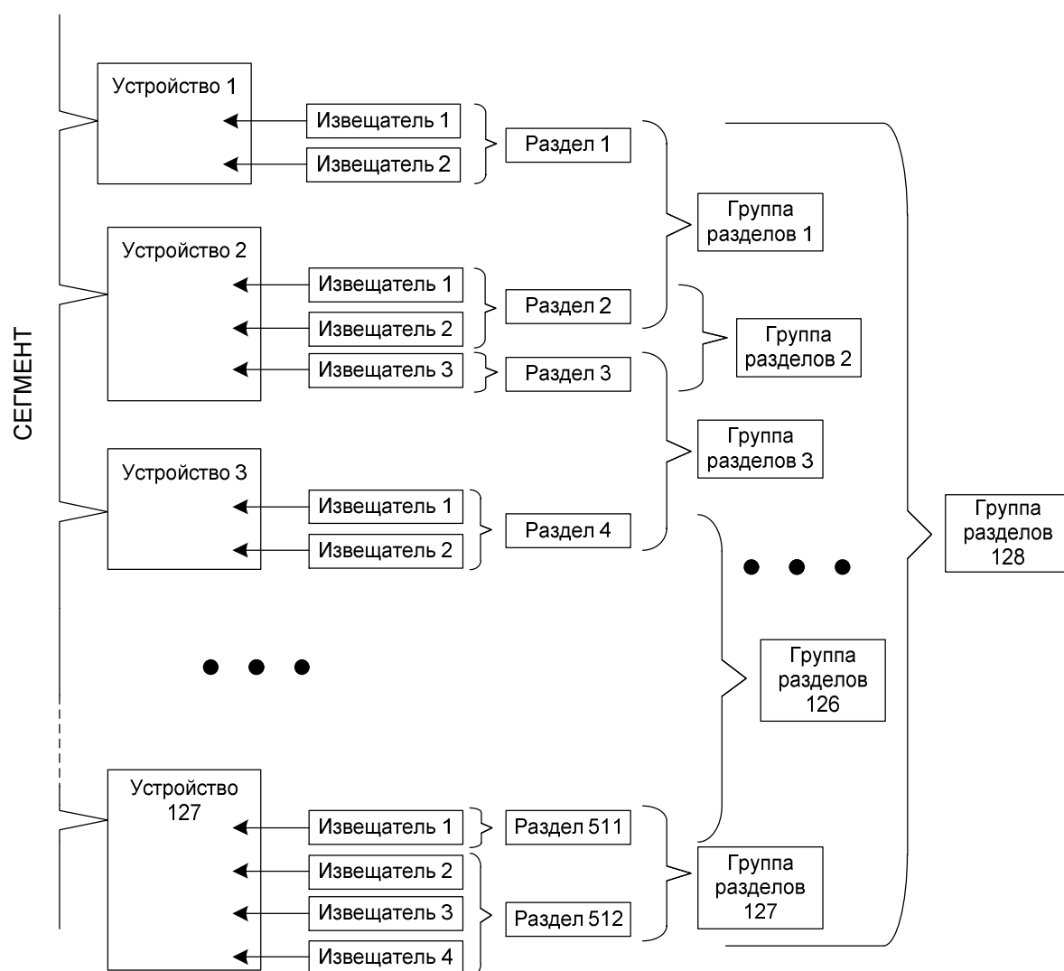
Рисунок 13 Принципы организации разделов и групп разделов
