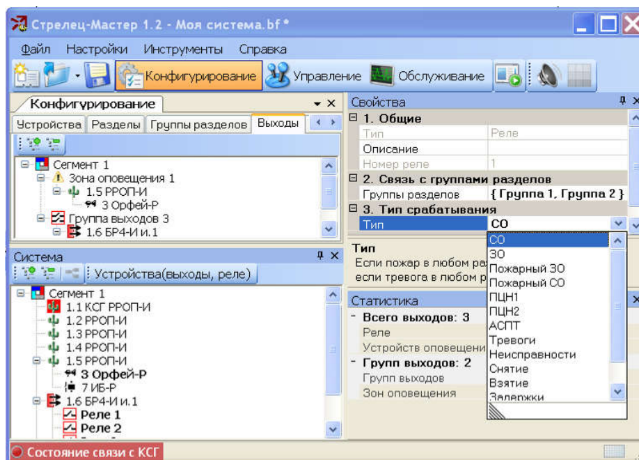
Рисунок 27 Конфигурирование событийных условий срабатывания выходов
