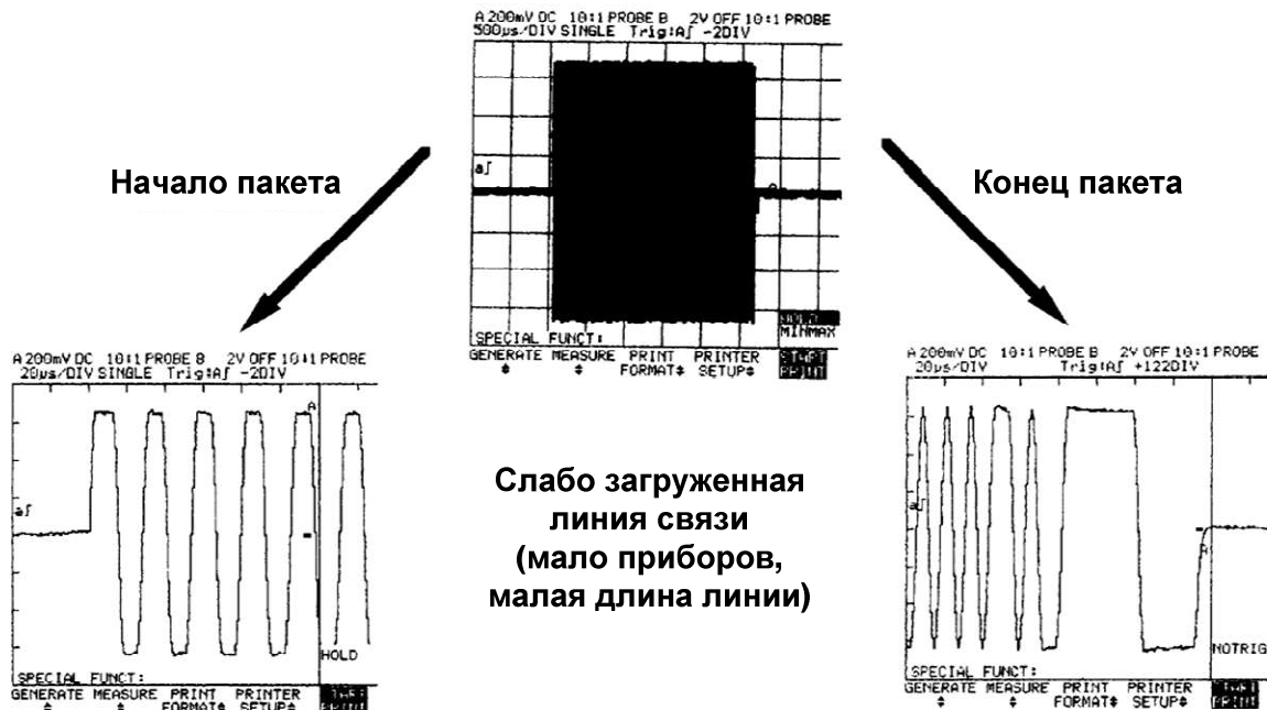
Рисунок 32 Типичная осциллограмма сигнала при слабой нагрузке линии связи
