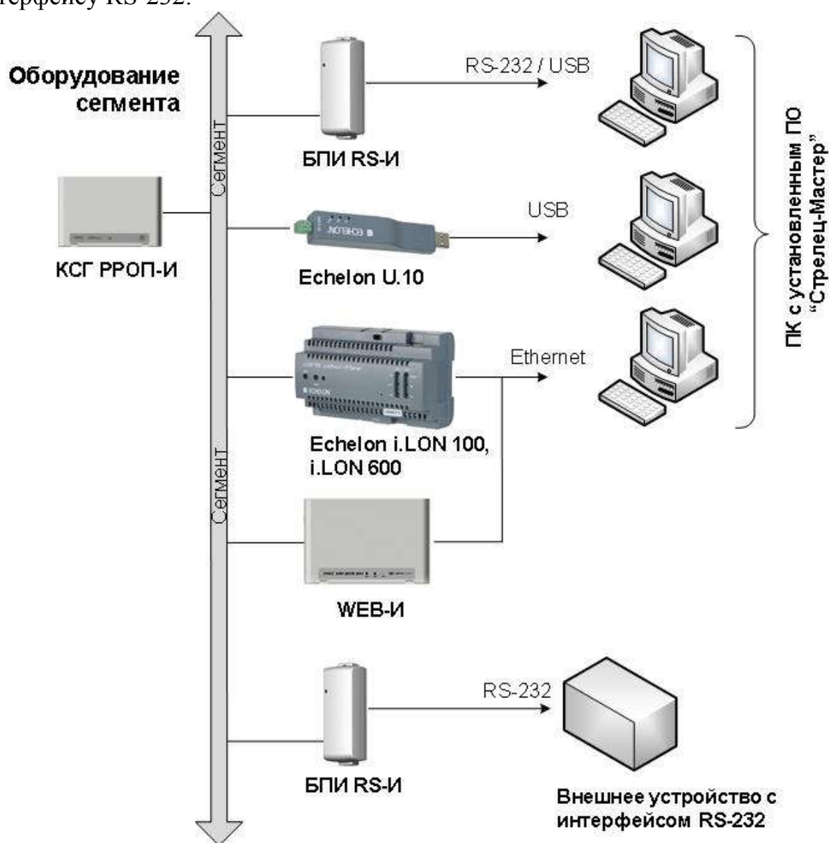
Рисунок 11 Блоки сетевых интерфейсов в ИСБ
