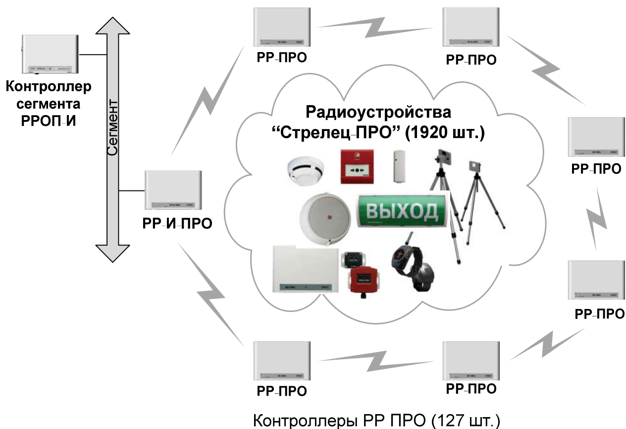
Рисунок 8 Радиоканальные устройства "Стрелец-ПРО"
