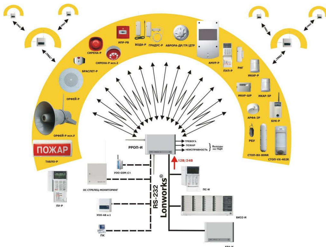
Рисунок 7 Радиосистема “Стрелец”
