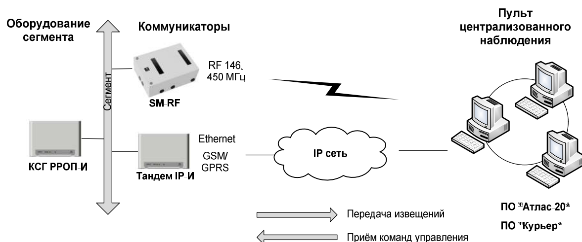
Рисунок 10 Коммуникационные устройства ИСБ
