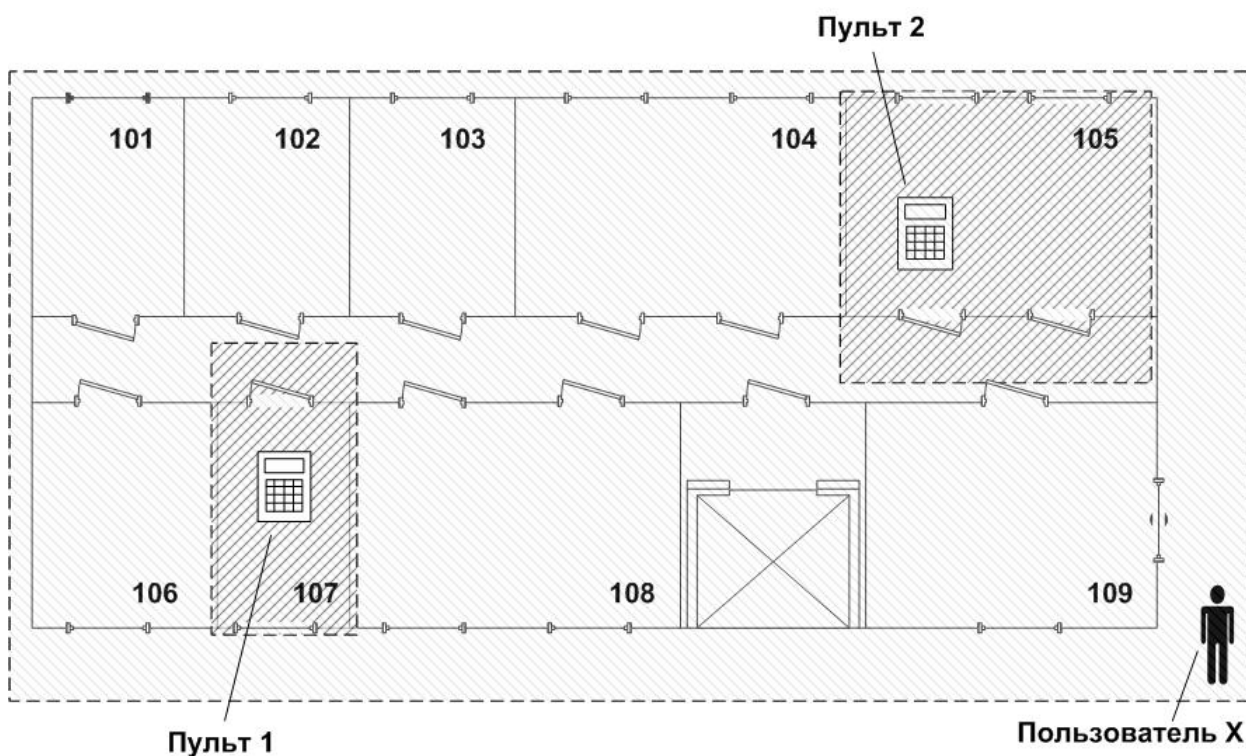
Рисунок 9 Права устройств управления по разделам
