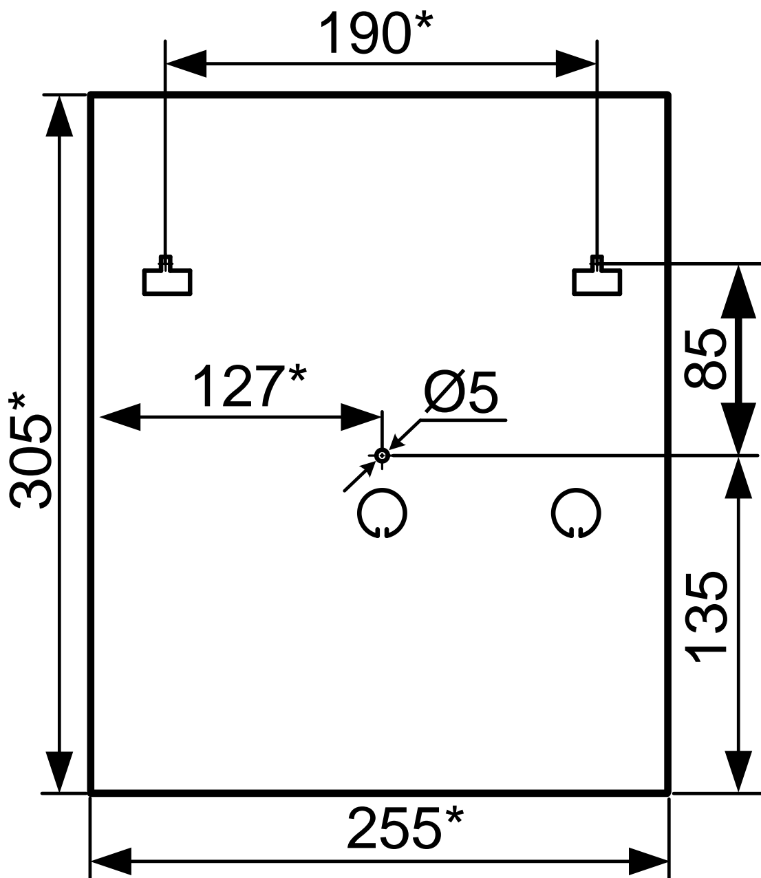
Габаритно-установочные размеры РИП
