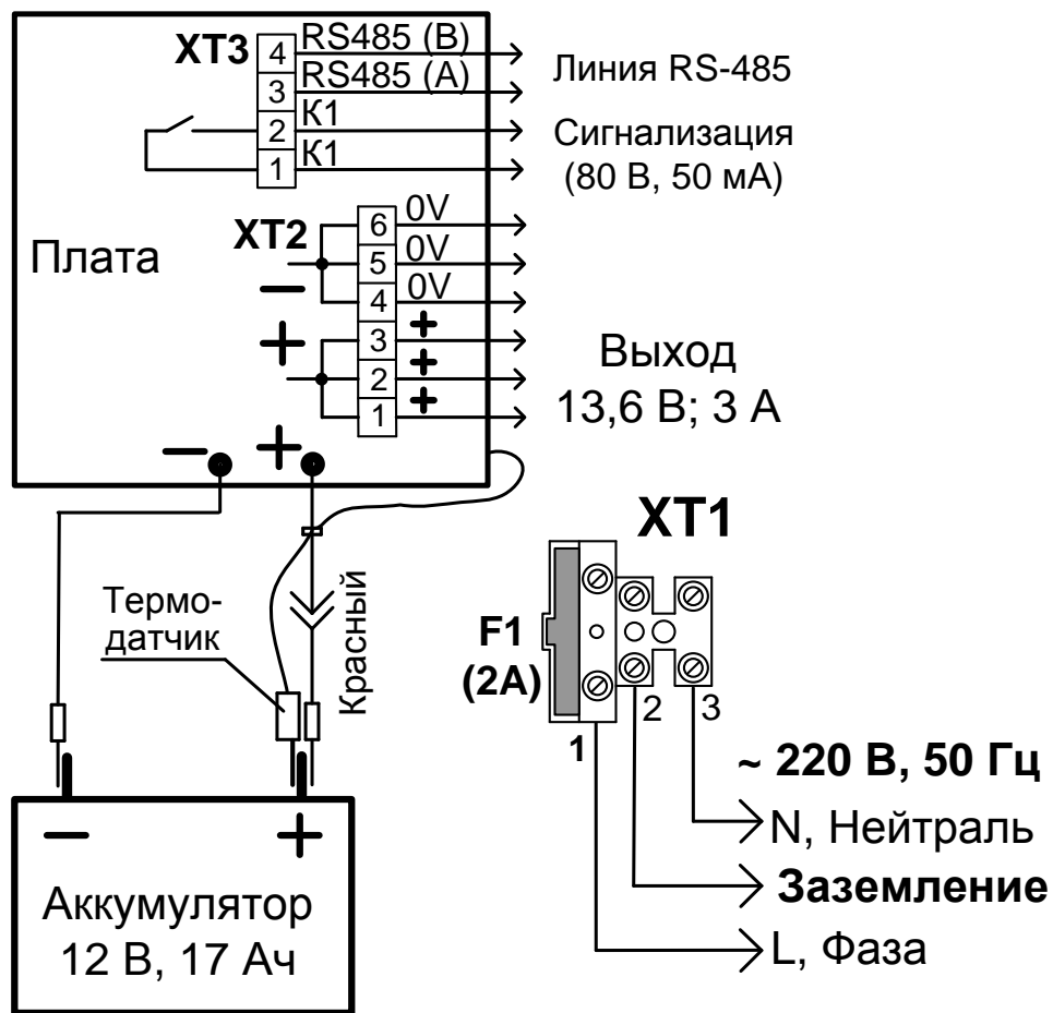
Схемы внешних подключений
