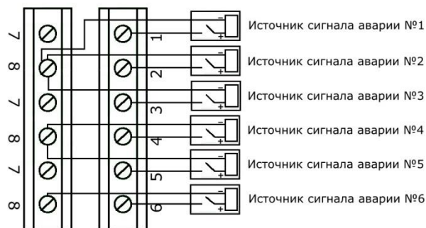
Рисунок 6. Подключение сигнальных линий при использовании подачи напряжения
