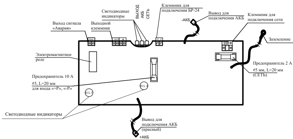
Рисунок 1 – Плата источника
