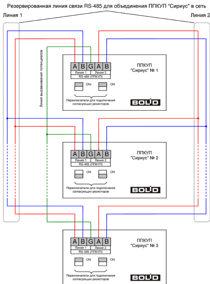
Рисунок 62. Схема объединения приборов «Сириус» в сеть
