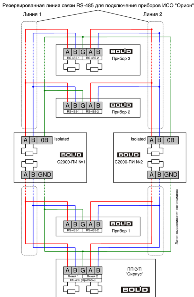
Рисунок 60. Схема подключения повторителей резервированного интерфейса RS-485 «С2000-ПИ»
