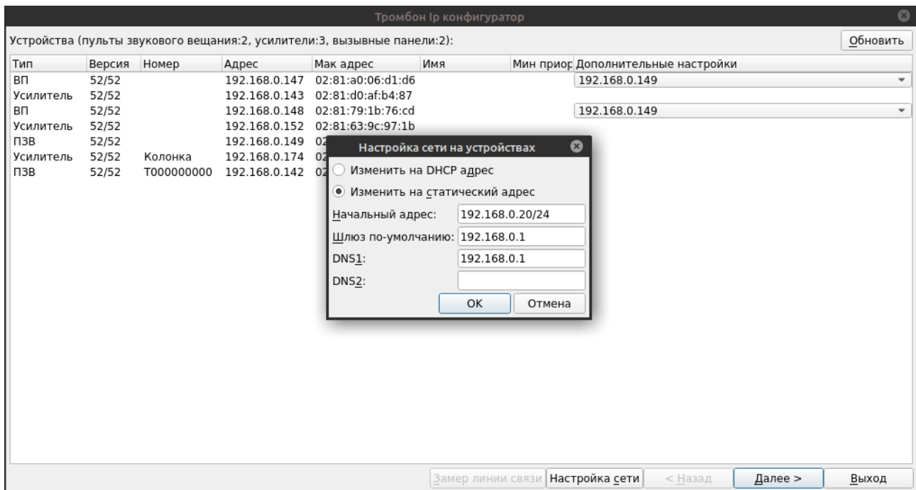
Рисунок 4: Настройка сети
