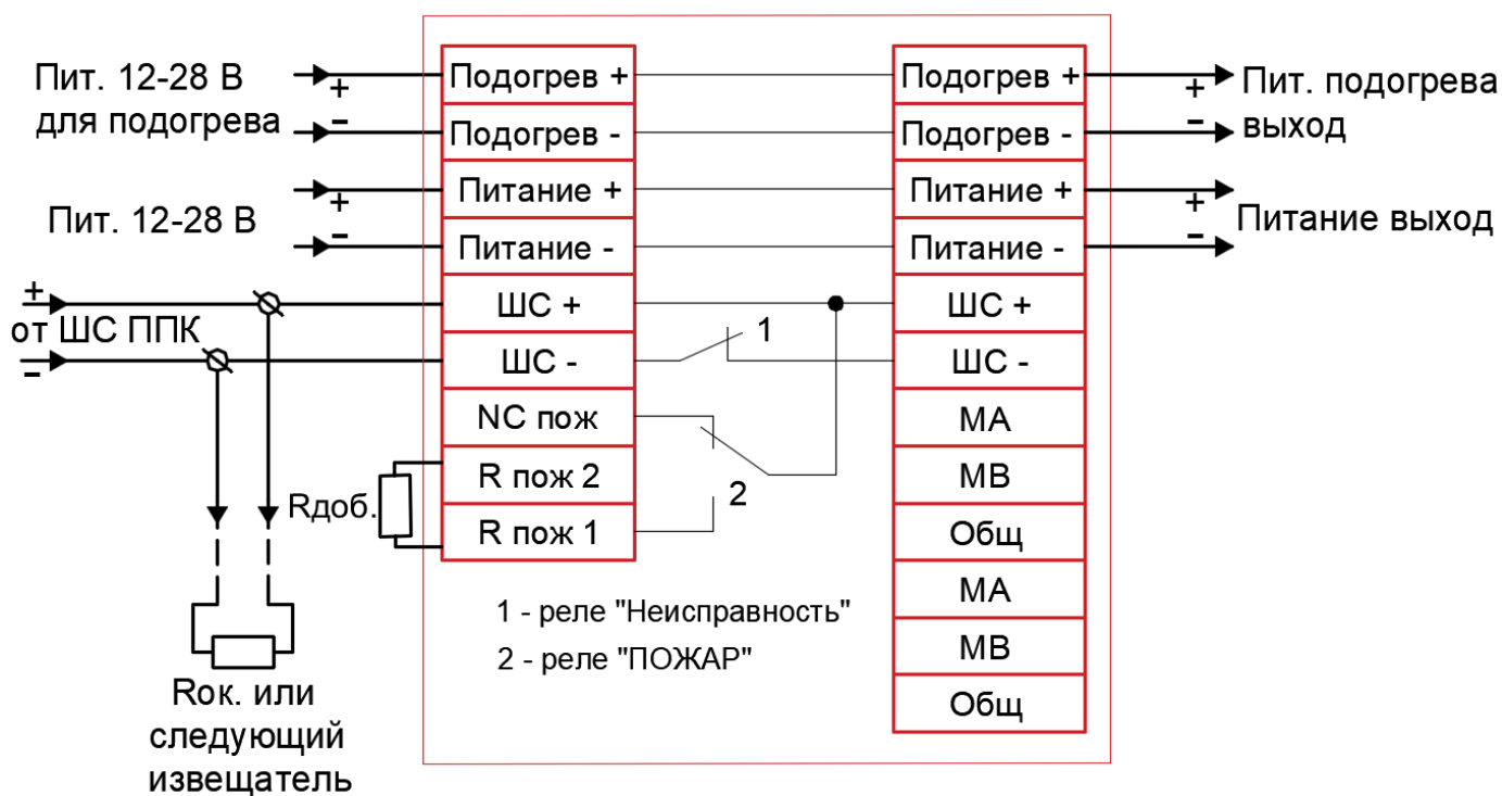
Рисунок 19 – Схема подключения к C2000-AP2 (AP-8) без использования режима «НЕИСПРАВНОСТЬ»
