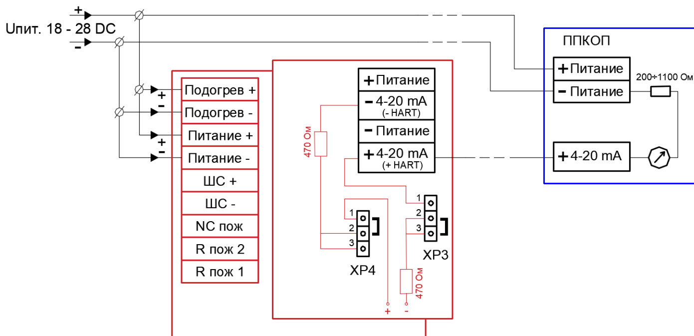
Рисунок 8 – Схема подключения извещателя с выходом 4-20 мА. (джампер XR3 в положении 2-3, джампер XR4 в положении 1-2)
