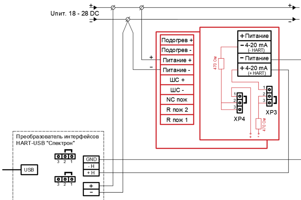
Рисунок 9 – Схема подключения 4-х проводная без использования режима «Неисправность»
