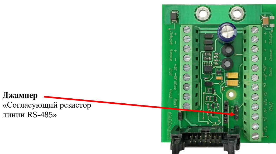
Рисунок 12 – Клеммная плата извещателя
