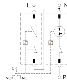
Рис. 2. Электрическая схема главного контура
