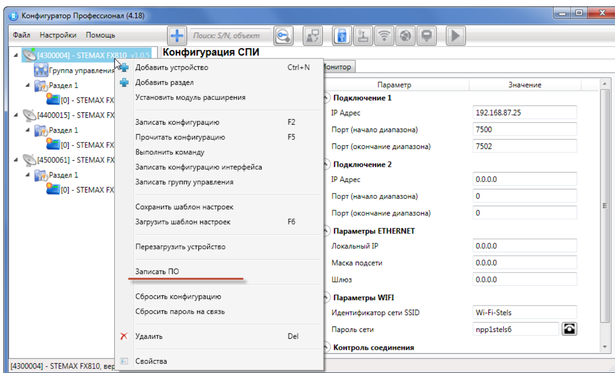
Рис. 13.1. Контекстное меню контроллера, выбор функции Записать ПО
