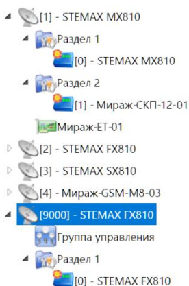
Рис. 5.3. Дерево устройств, частично свернуто
