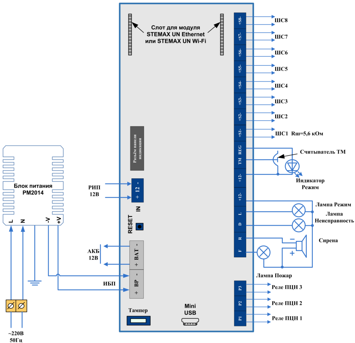
Схема внешних подключений ППКОП STEMAX FX810
