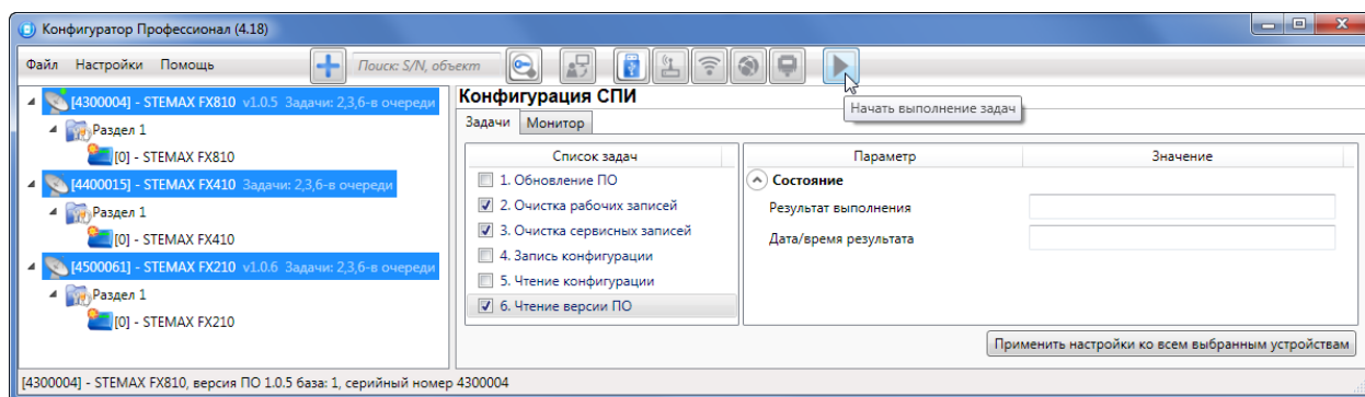
Рис. 8.5. Вкладка Задачи
