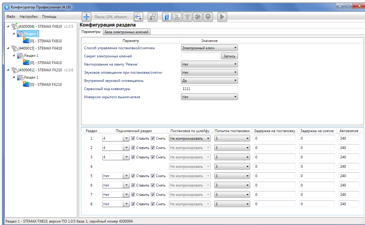
Рис. 9.3. Пример 1
