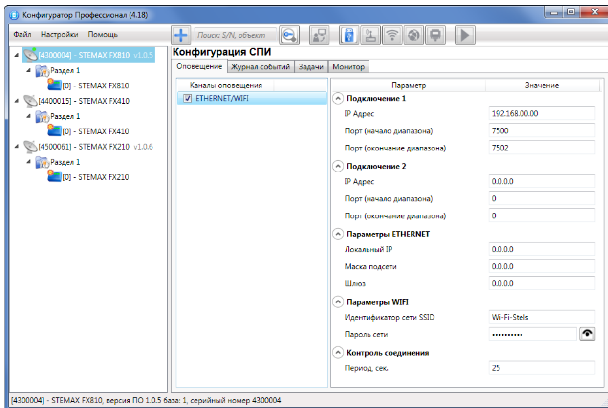
Рис. 8.2. Вкладка Оповещение
