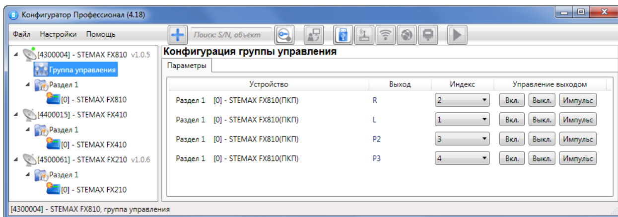
Рис. 11.2. Параметры и элементы дистанционного управления
