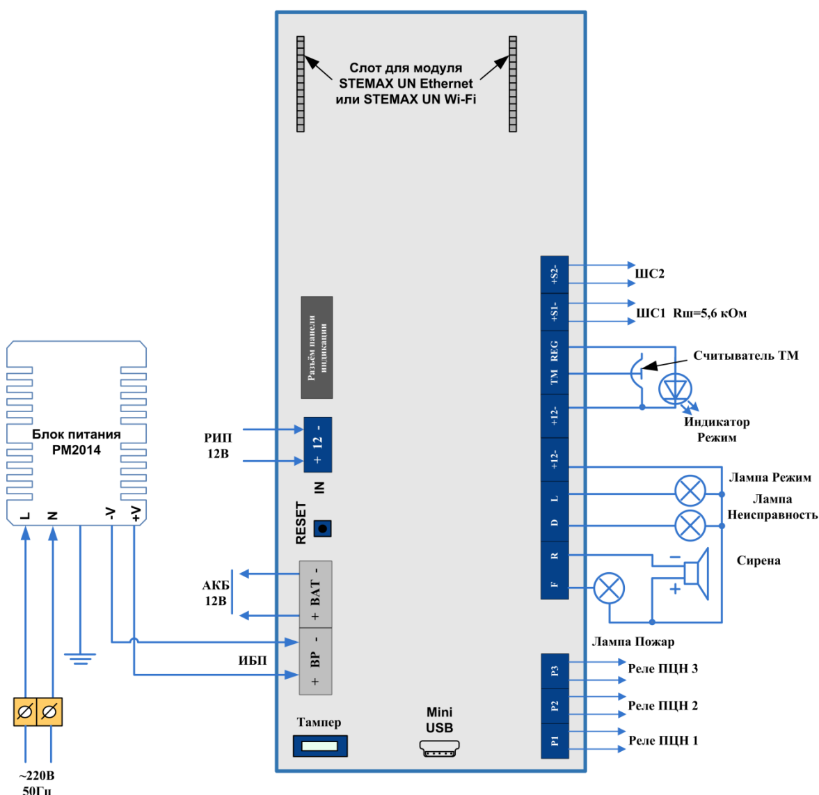
Схема внешних подключений ППКОП STEMAX FX210
