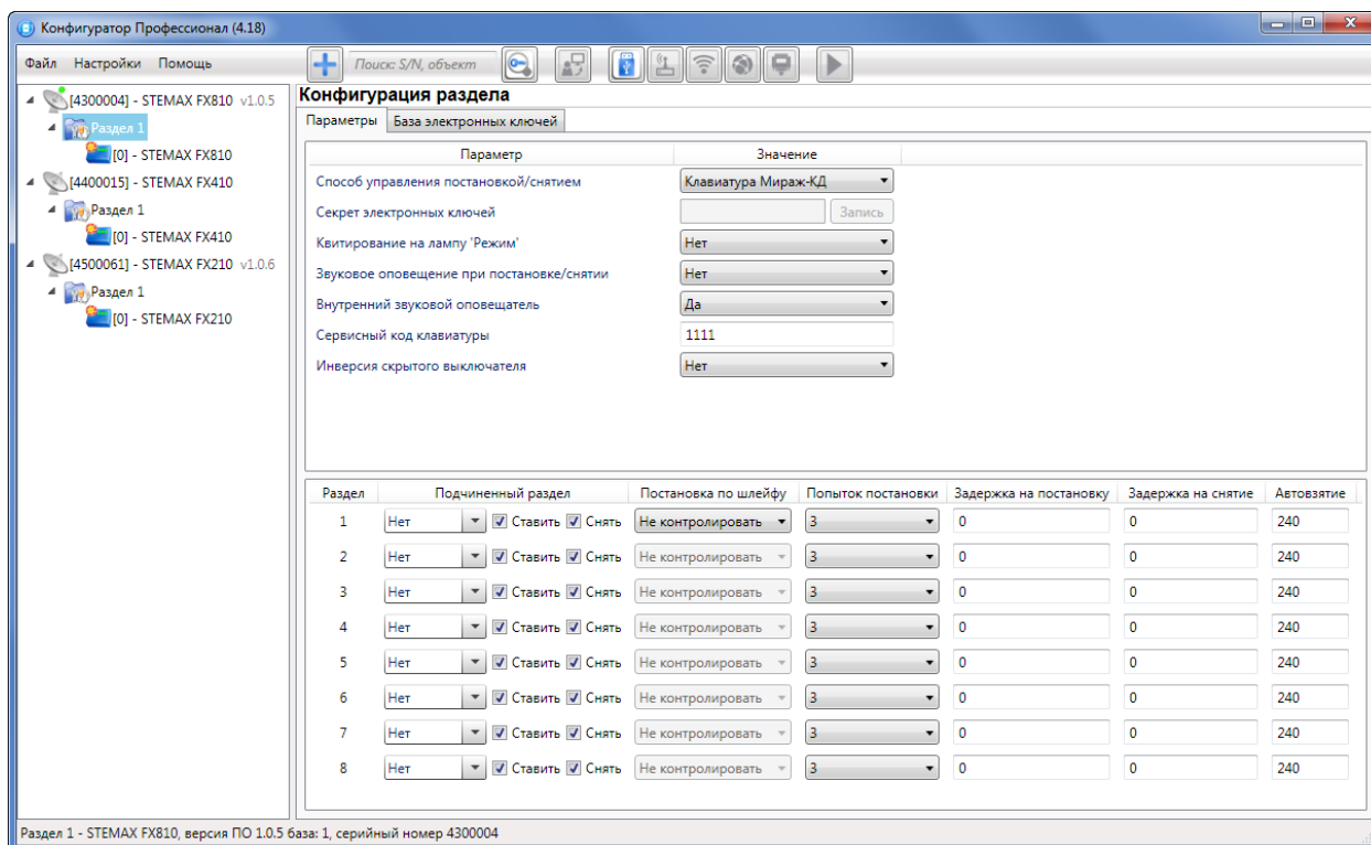
Рис. 9.2. Вкладка Параметры
