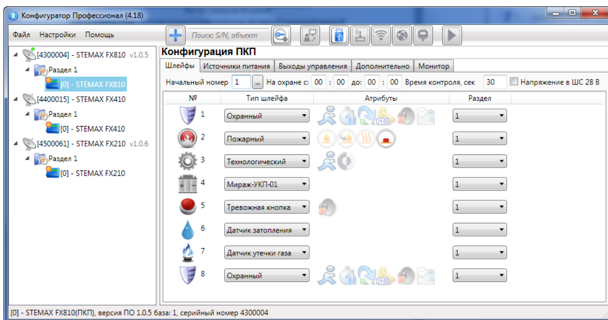
Рис. 10.2. Вкладка Шлейфы
