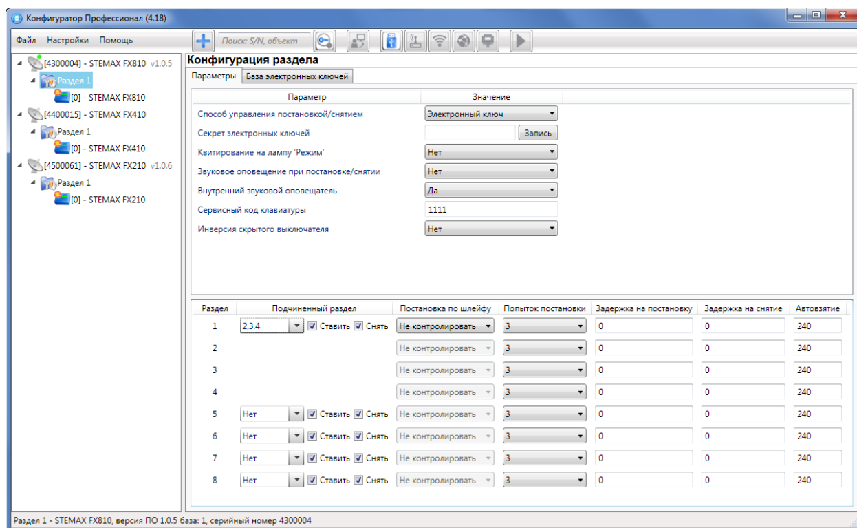
Рис. 9.4. Пример 2
