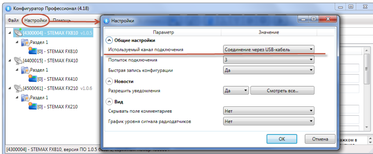
Рис. 6.1. Окно Настройки
