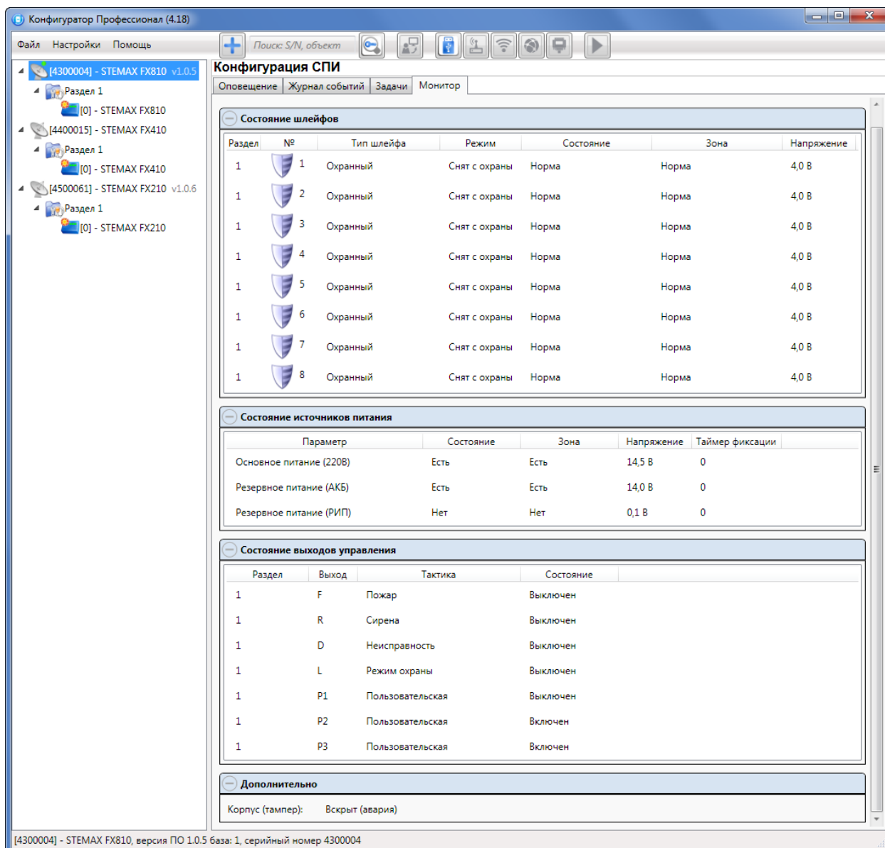
Рис. 8.6. Вкладка Монитор
