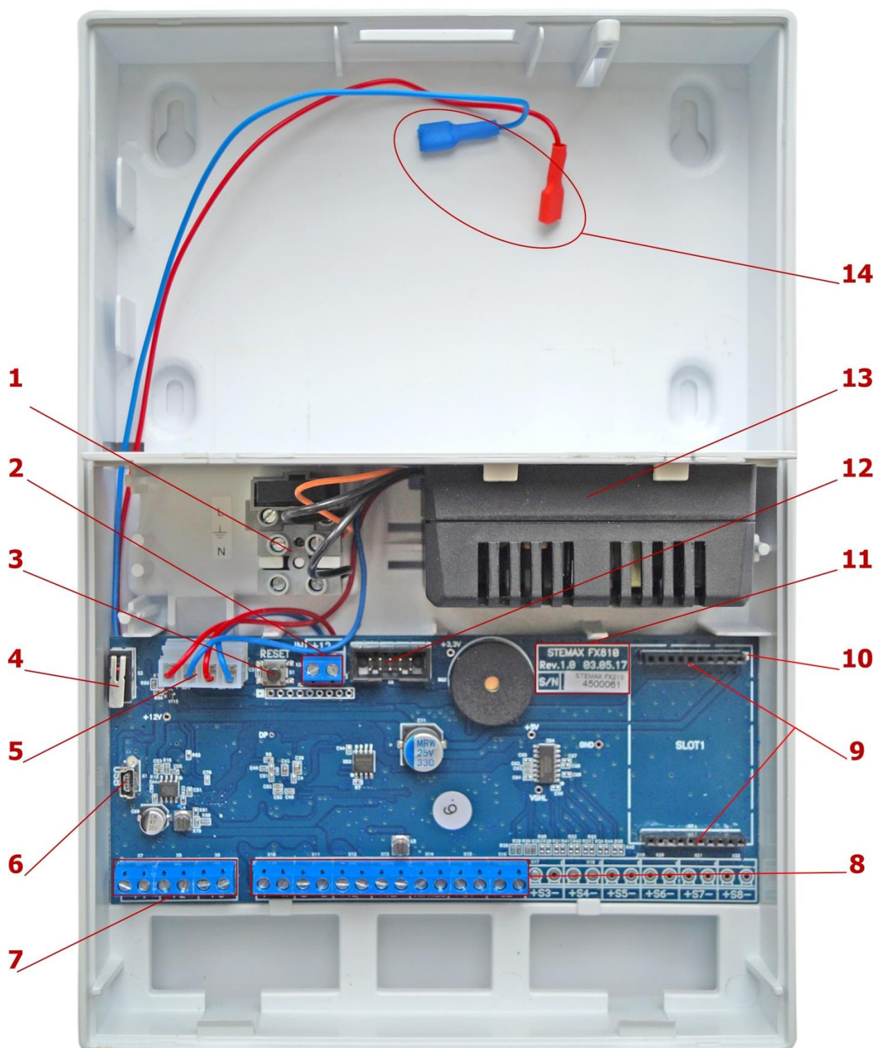
Вид ППКОП STEMAX FX210 со снятой крышкой
