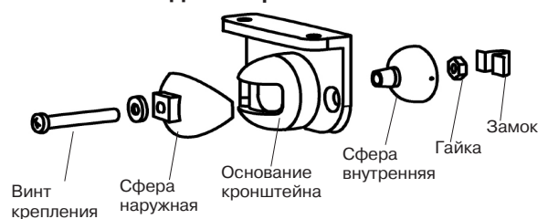
Рисунок 3 - Кронштейн
