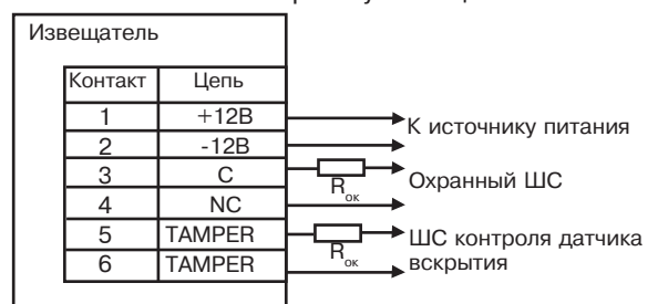
Рисунок 4 - Схема подключения
