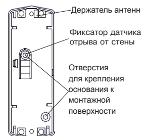
Рисунок 2 – Основание
