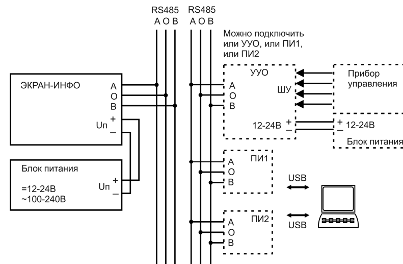
Рисунок 7. Схема соединений ЭКРАН-ИНФО-RGB, УВО-RGB, ПИ1 и ПИ2.
