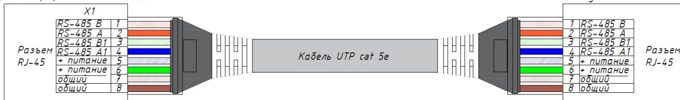
Рисунок 14. Схемы подключения кабеля от БС/БУ или коммутационной коробки к МП.
