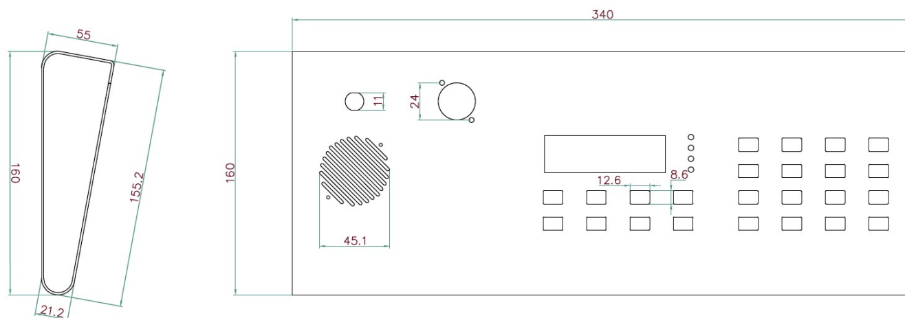
Рисунок 2. Габаритные размеры МП МЕТА 18740-16
