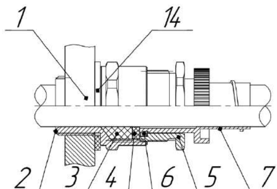
г) Прокладка кабеля в металлорукаве
