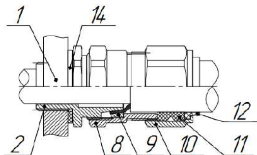
д) Прокладка бронекабеля
