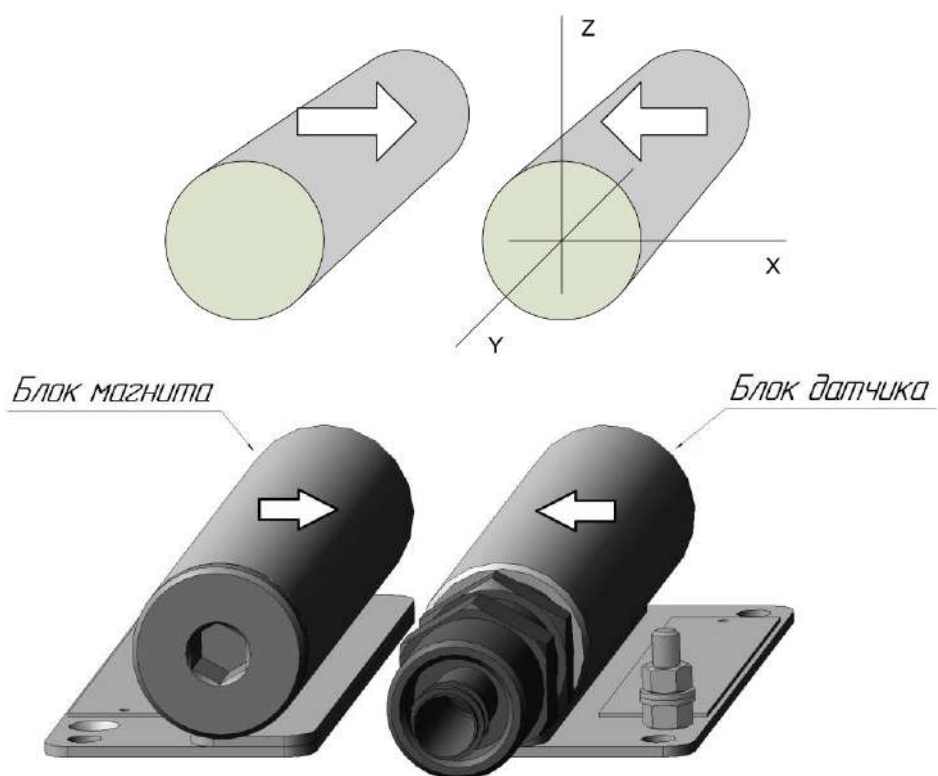
Рис. 4. Схема расположения и относительного перемещения блоков датчика и магнита.
