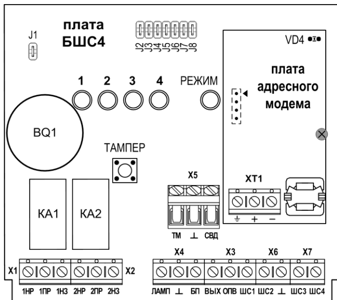
Рис.10 Плата БШС4
