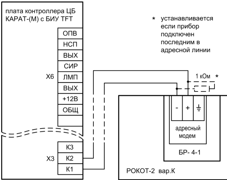
Рис.А15 Схема подключения Рокот-2 вар.К к ЦБ
