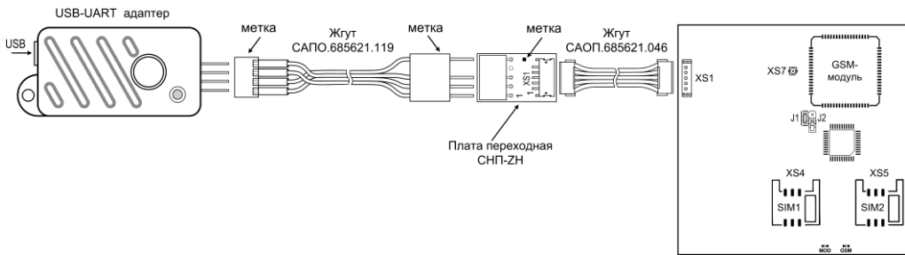
Рис.А19 Подключение USB-UART адаптера к универсальному коммуникатору
