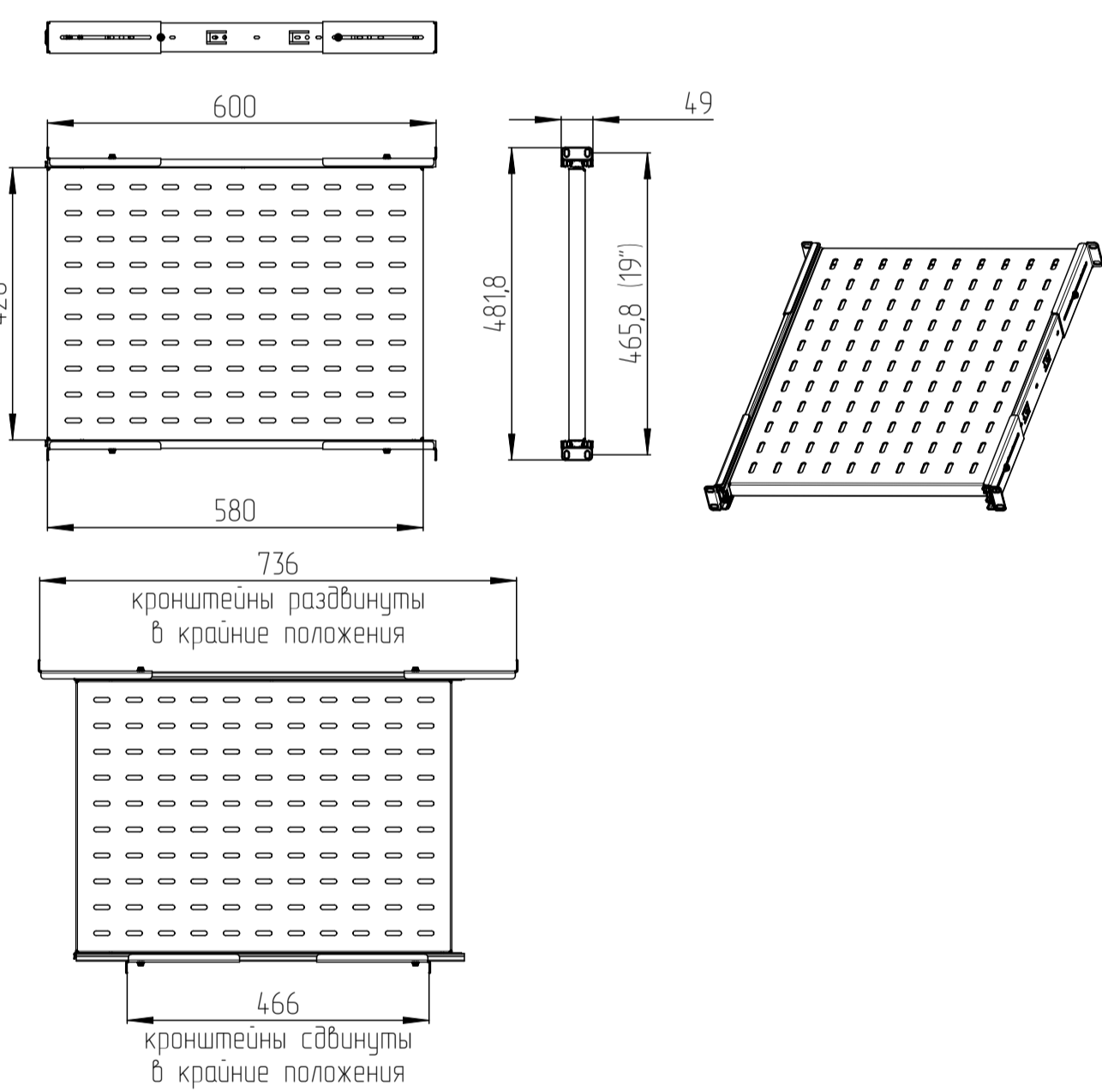
Полка ТСВ-45
