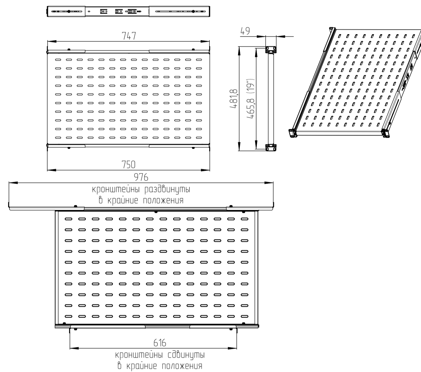
Полка ТСВ-К4
