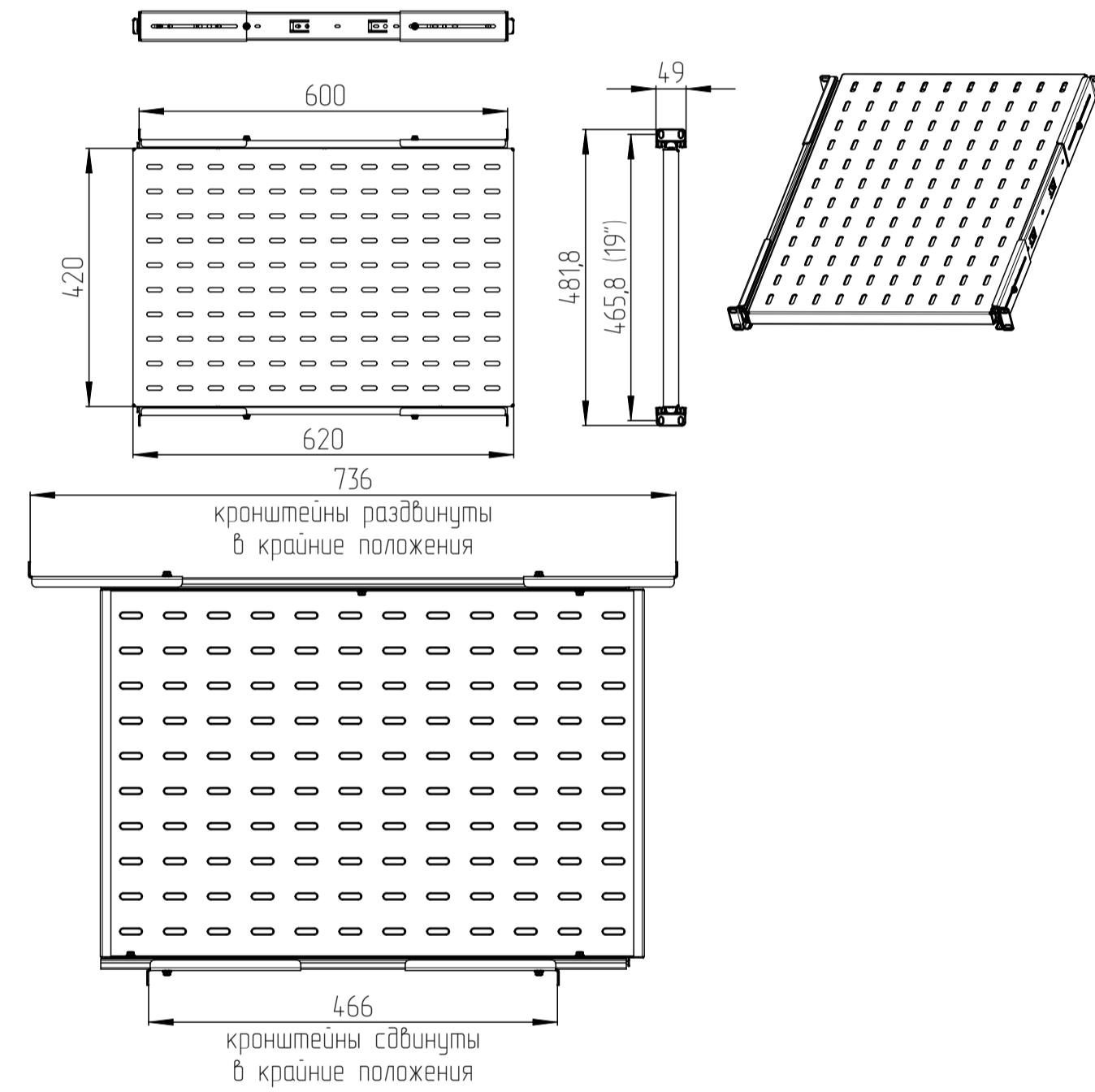
Полка ТСВ-КС
