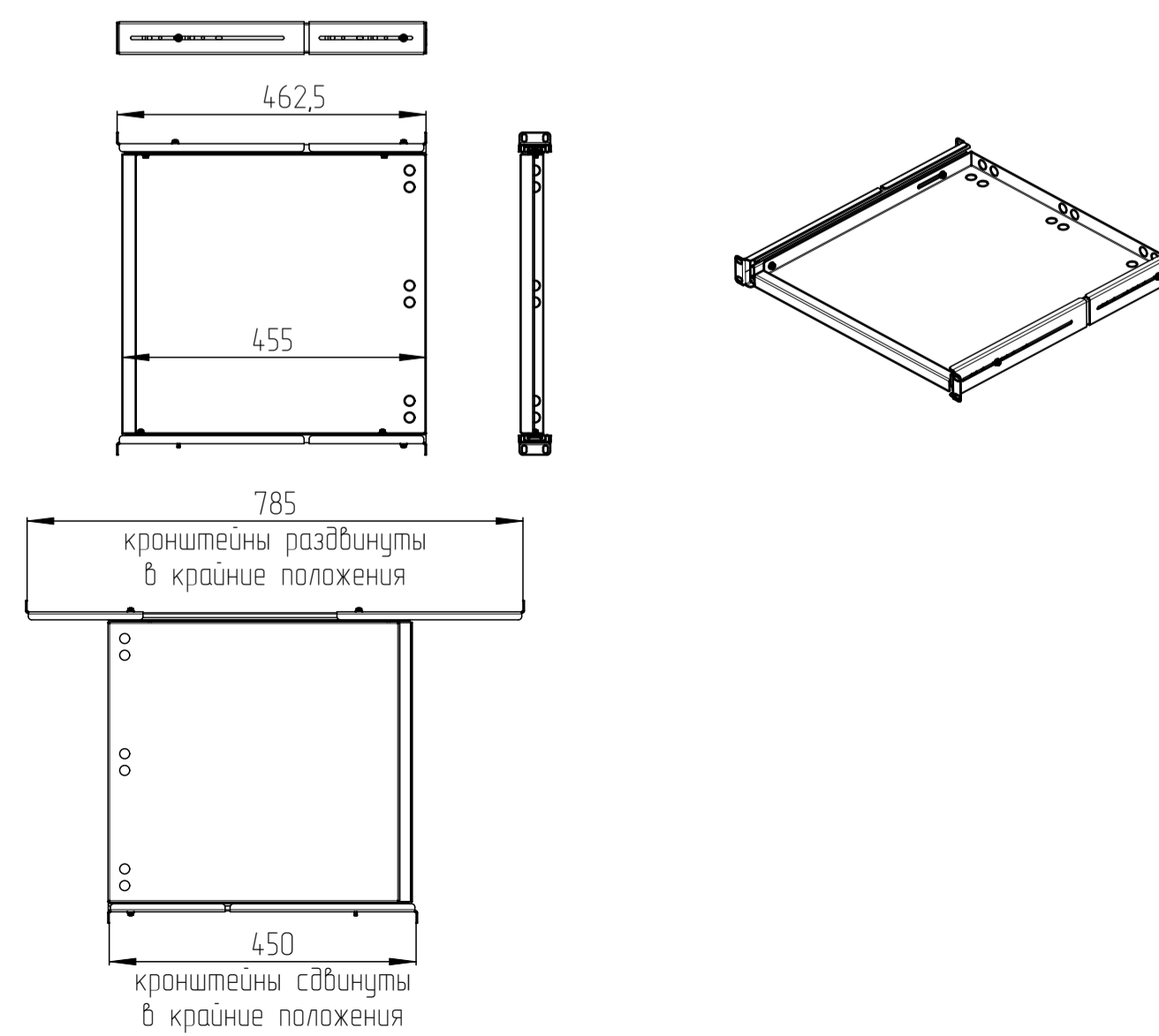
Полка ТСВ-К4
