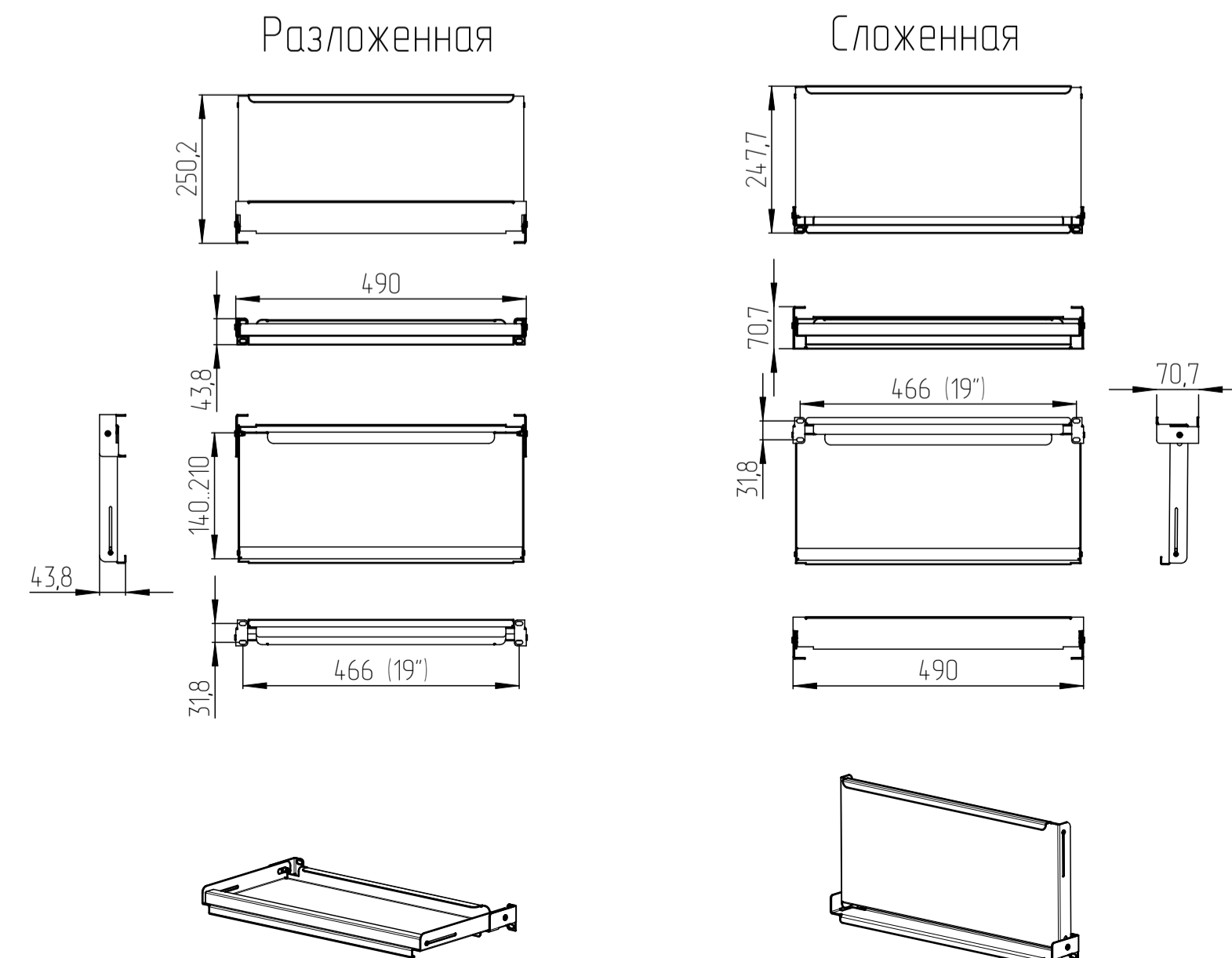
Полка ТСВ-КС
