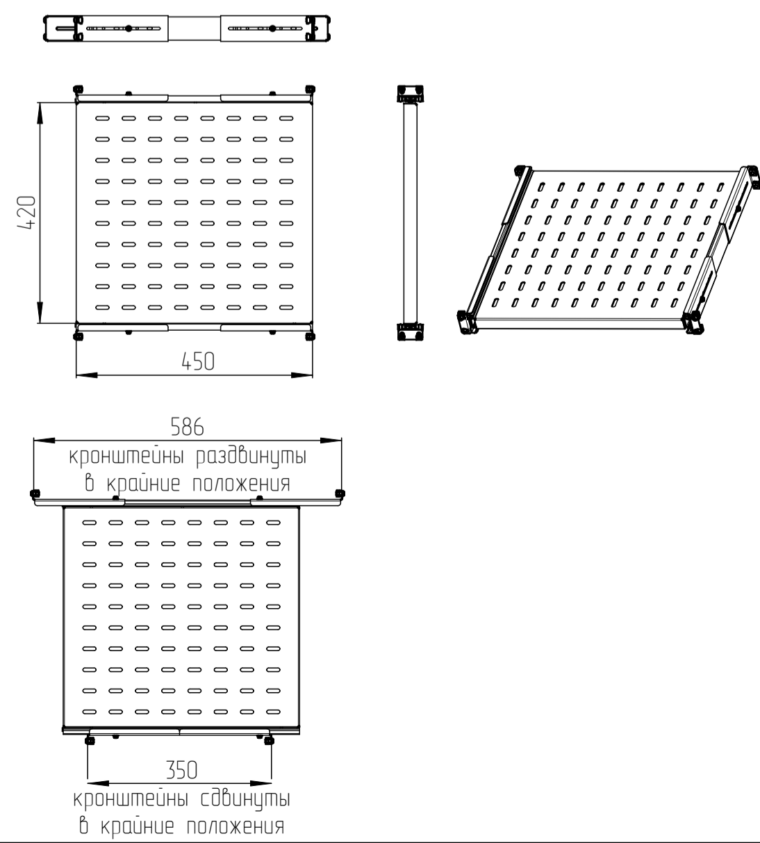
Полка ТСВ-45
