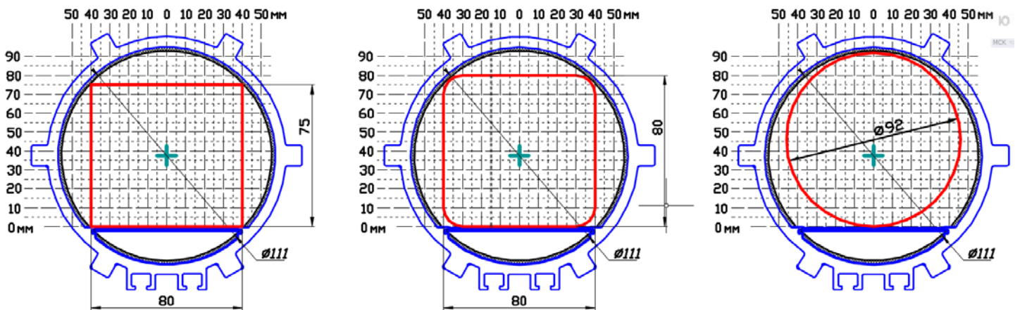
Рисунок А2 – Сечение термокожуха, мм
