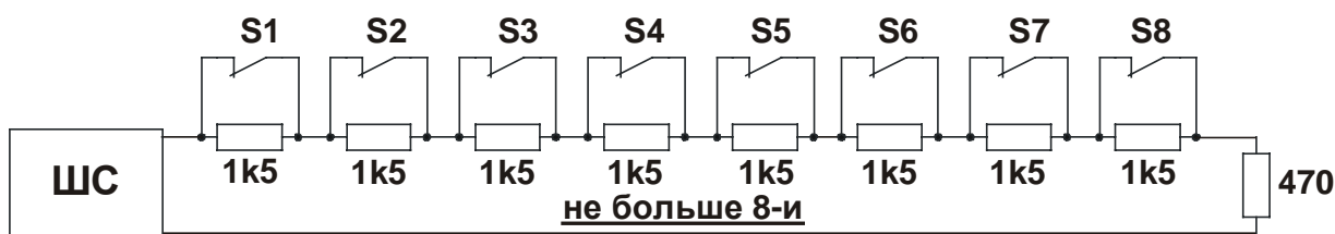
Рис. Схема 7 Последовательное подключение нескольких НЗ извещателей.
