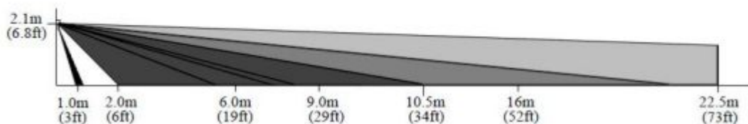
Рис. 6 Диаграмма зоны обнаружения SKAU-01-Ш
