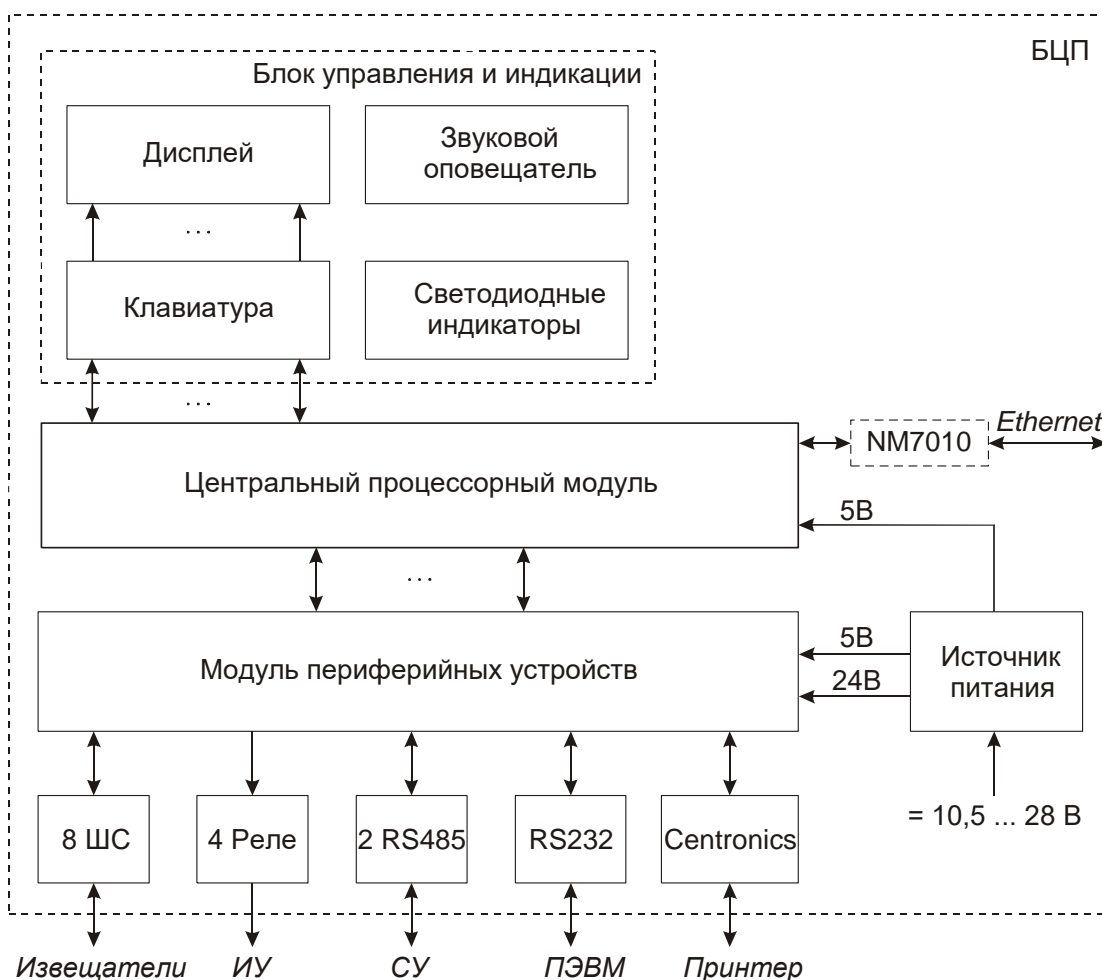
Рис. 2 Электрическая структурная схема БЦП Р-08 исп. 2
