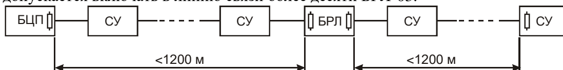
Рис. 13 Использование БРЛ-03 для удлинения линии связи
