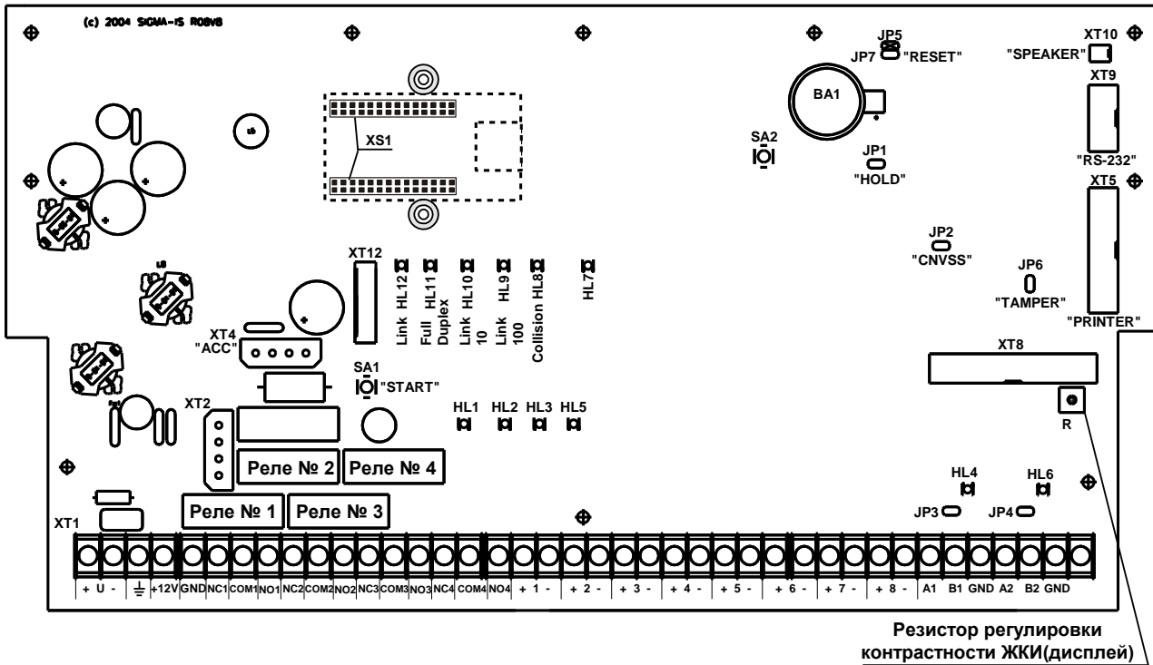
Рис. 31 Плата БЦП исп. 2,3
