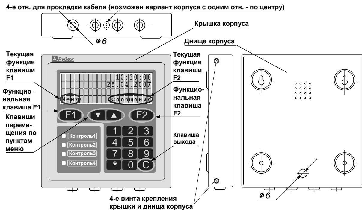
Рис. 11 БЦП исп.6 (IP20)
