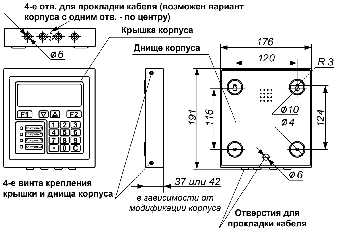
Рис. 41 Габаритные и присоединительные размеры БЦП исп. 6 (IP20)
