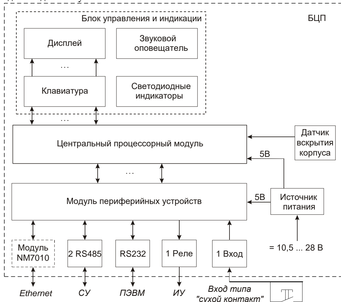
Рис. 6 Электрическая структурная схема БЦП Р-08 исп. 6
