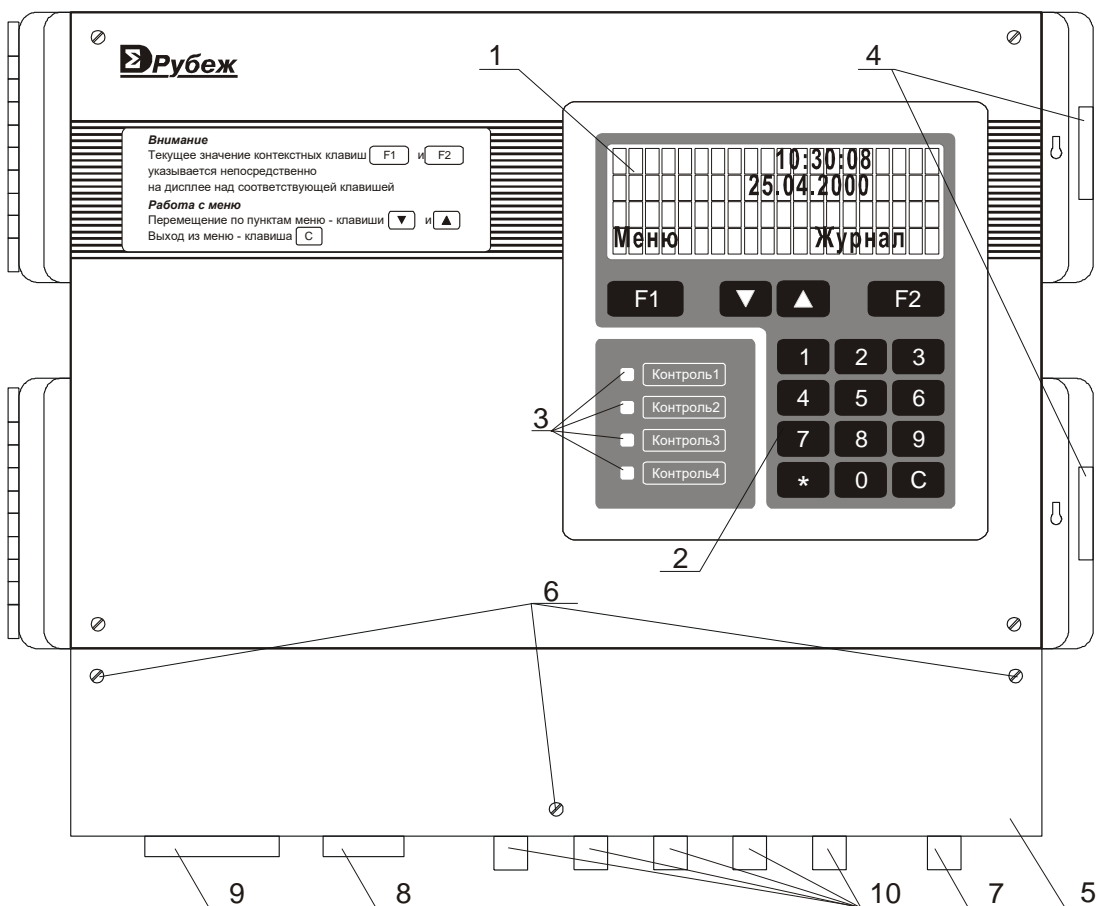
Рис. 7 Внешний вид БЦП (исп. 2)
