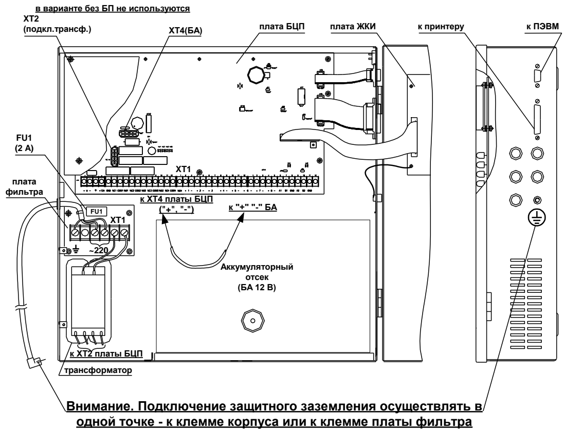
Рис. 29 Расположение элементов БЦП исп. 3
