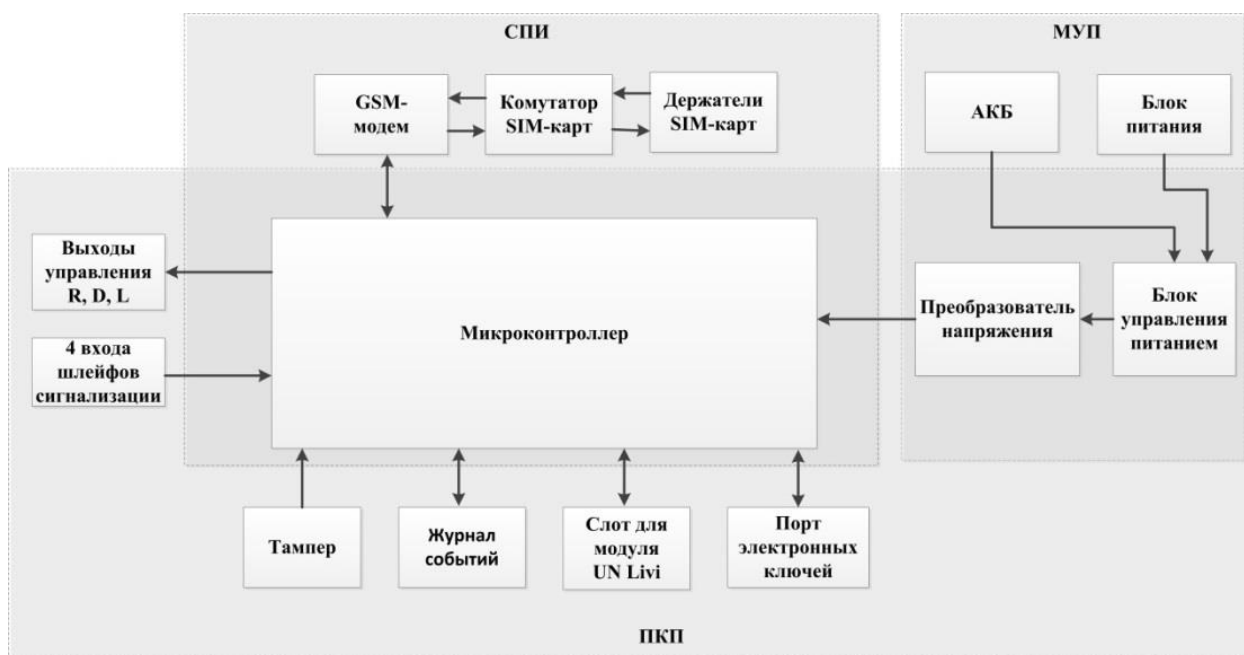
Рисунок 5.1 — Функциональная схема
