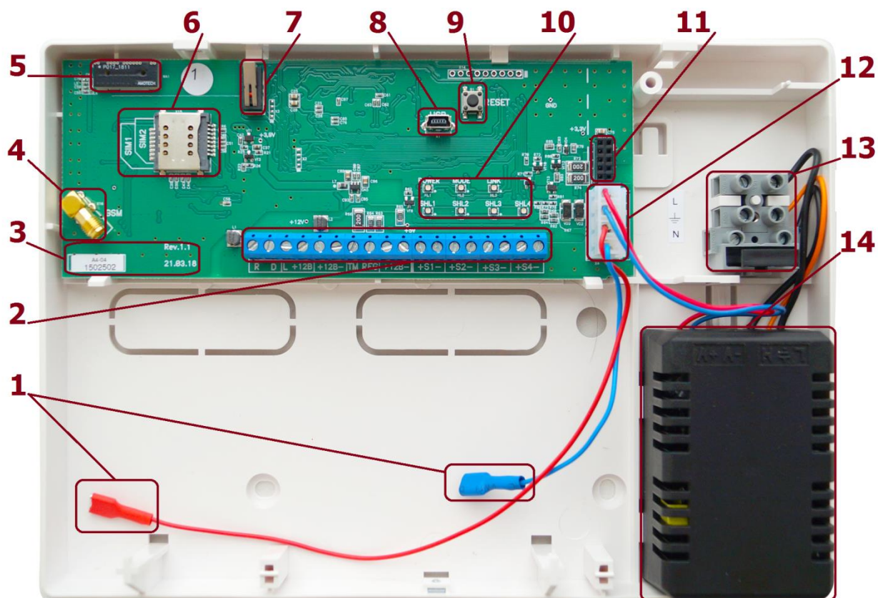
Рисунок А.0.1 – Вид контроллера со снятой крышкой
