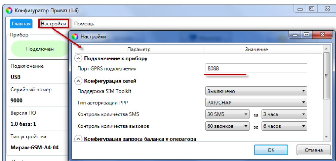
Рисунок 7.13 – Изменение номера TCP/IP-порта для GPRS-подключения
