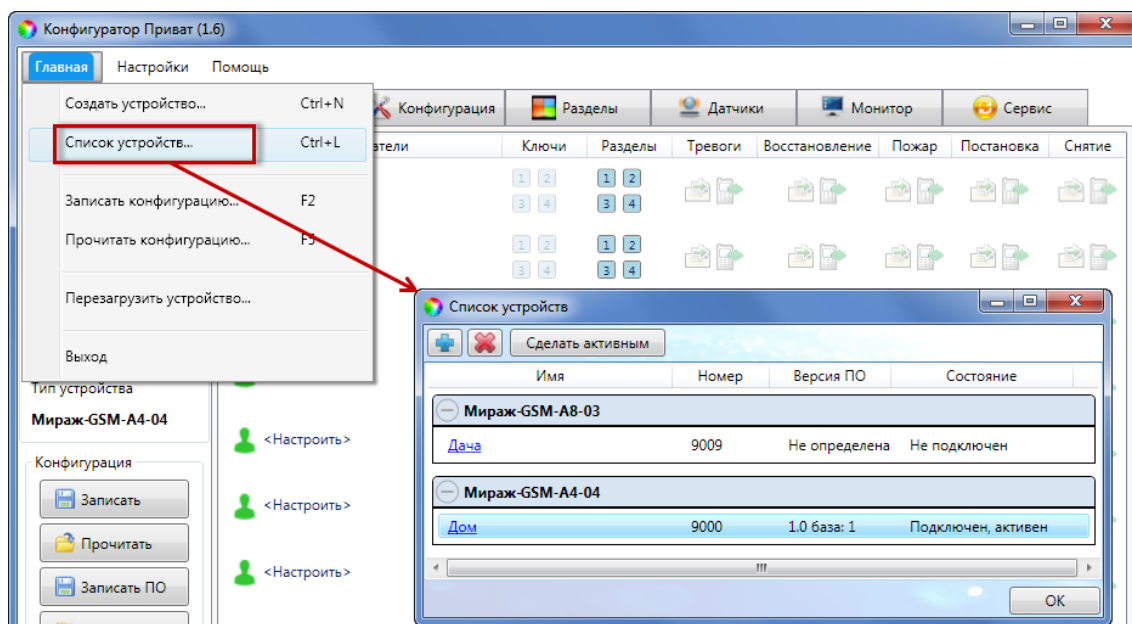
Рисунок 7.12 – Окно Список устройств
