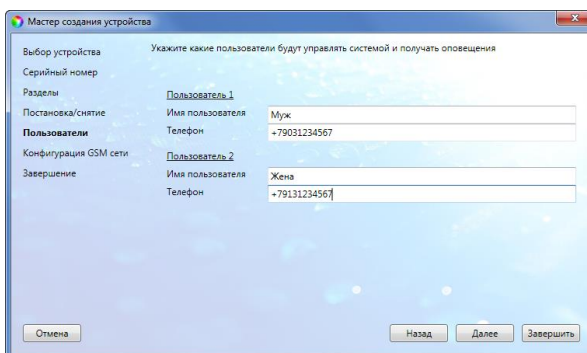
Рисунок 7.8 — Окно Пользователи
