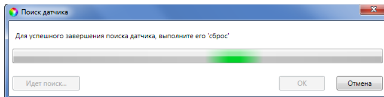
Рисунок 7.42 — Поиск радиоустройства
