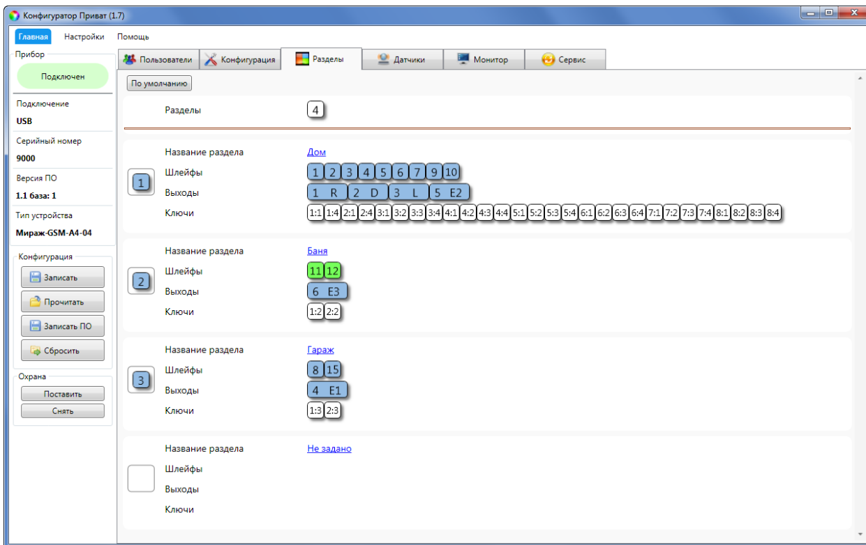
Рисунок 7.36 — Пример конфигурации
