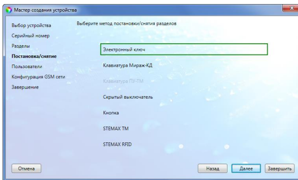
Рисунок 7.7 — Окно Постановка/снятие
