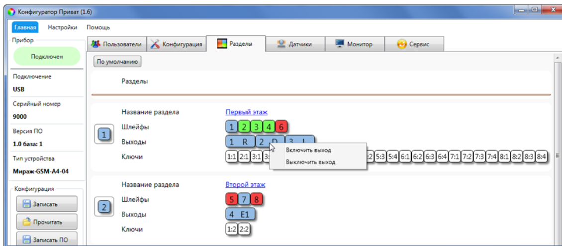
Рисунок 7.38 — Управление выходами
