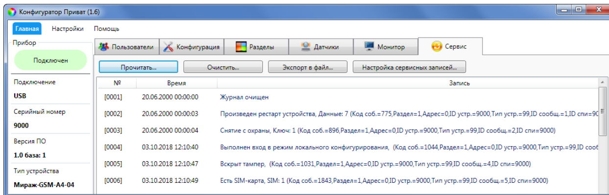
Рисунок 7.50 — Вкладка Сервис
