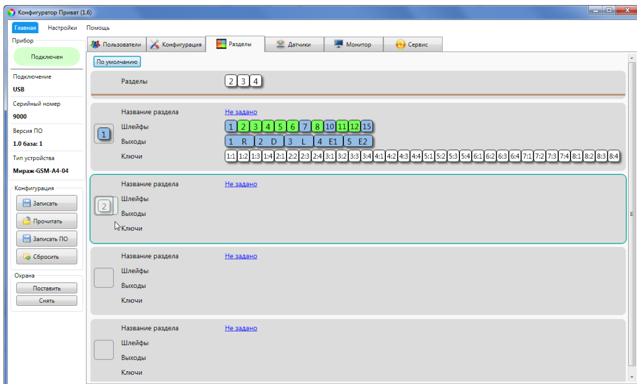
Рисунок 7.32 — Активация раздела 2
