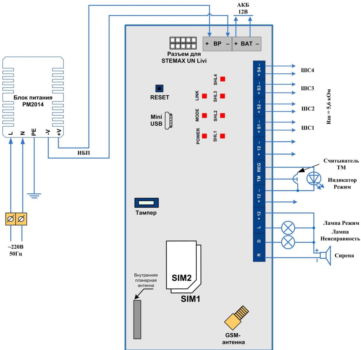
Рисунок Б.0.1 – Схема внешних подключений
