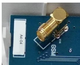
Рисунок 6.1 — SMA-разъем для подключения GSM-антенны
