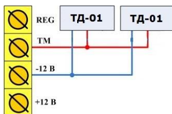
Рисунок 6.3 — Схема подключения цифровых датчиков температуры Мираж-ТД-01
