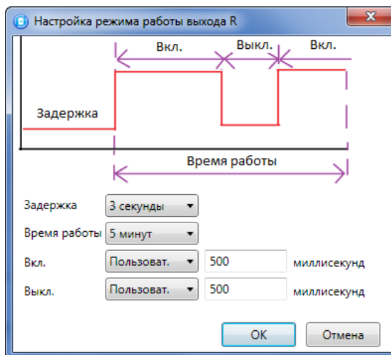
Рисунок 7.24 — Окно Настройка режима работы выхода
