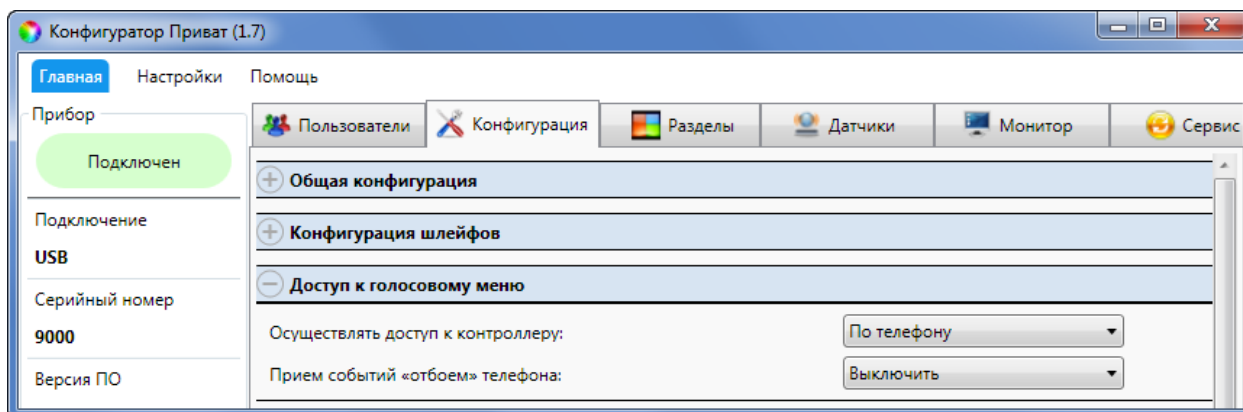
Рисунок 7.22 — Блок Доступ к голосовому меню
