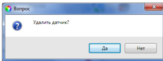
Рисунок 7.45 — Окно Вопрос
