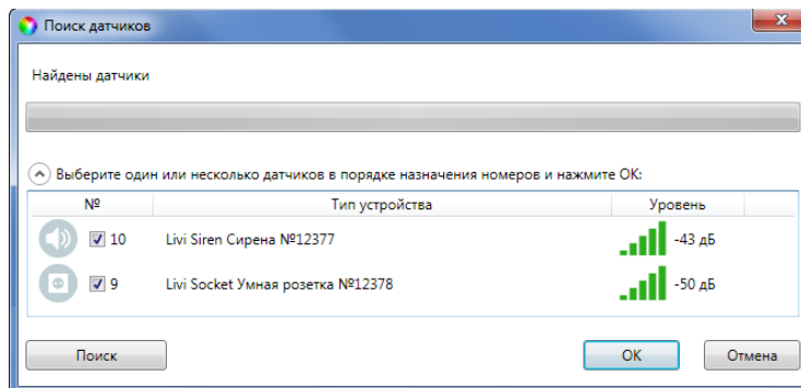
Рисунок 7.43 — Поиск радиоустройства
