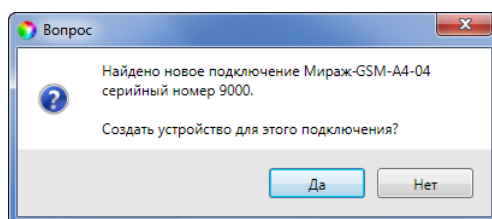
Рисунок 7.3 — Окно Вопрос
