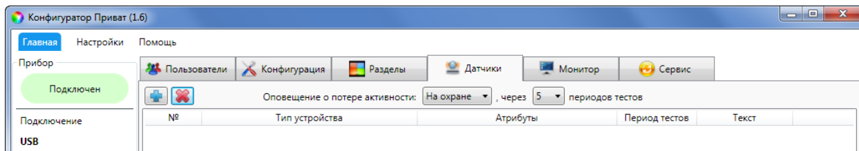
Рисунок 7.40 — Вкладка Датчики
