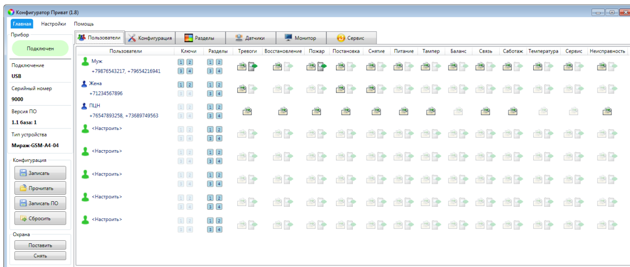
Рисунок 7.15 — Вкладка Пользователи
