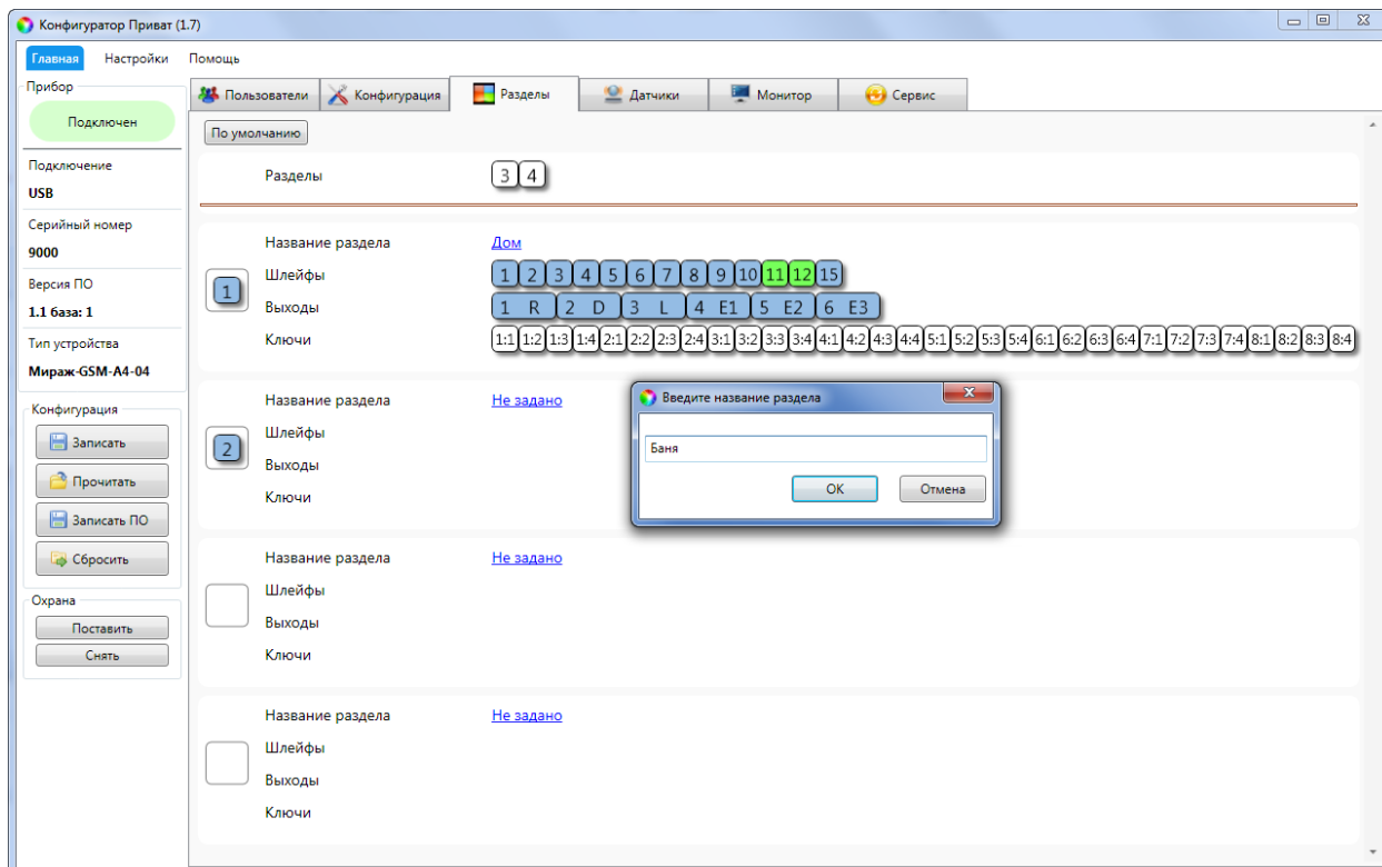
Рисунок 7.33 — Вкладка Разделы
