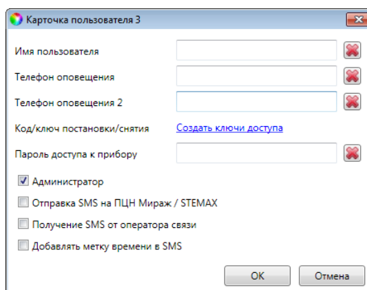
Рисунок 7.17 — Карточка пользователя
