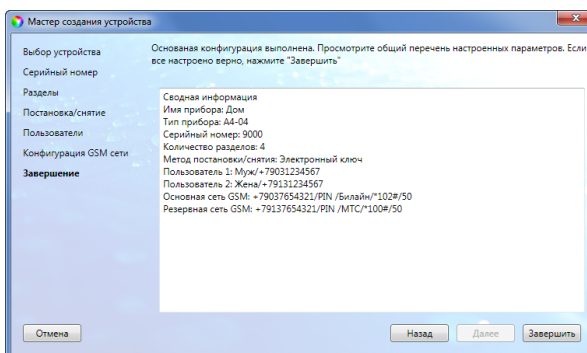
Рисунок 7.10 – Окно Завершение
