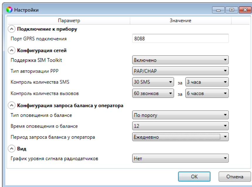
Рисунок 7.53 — Меню Настройки
