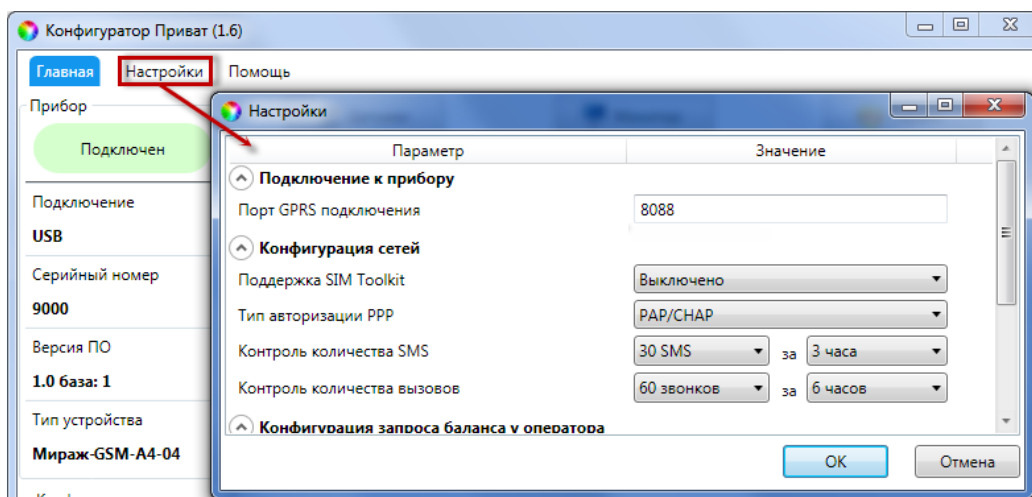
Рисунок 7.52 – Меню Настройки
