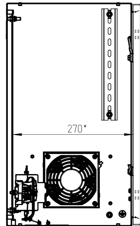
C-C 1:5
