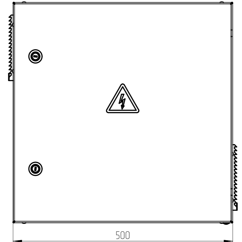
Вид спереди. Масштаб 1:5
