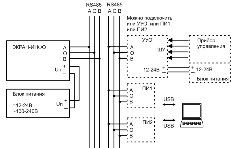
Рисунок 7. Схема соединений ЭКРАН-ИНФО-RGB, УВО-RGB, ПИ1 и ПИ2.
