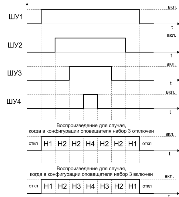
Рисунок 13. УЗО-RGB. Диаграмма выбора ШУ (Н – воспроизводимый набор).
