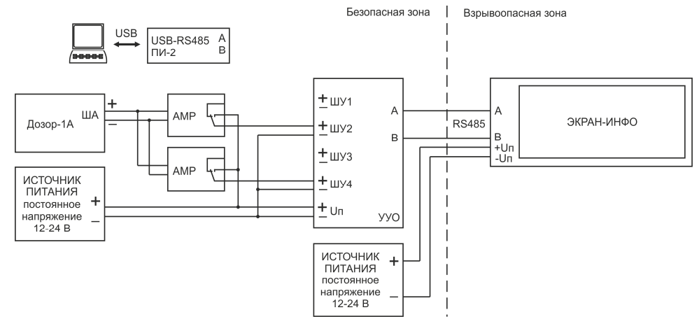
Рисунок 12. Пример подключения оповещателя ЭКРАН-ИНФО-RGB в адресный шлейф прибора Дозор-1А через адресные метки реле АМР и устройство управления УЗО-RGB.
