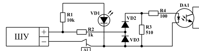
Рисунок 9. Схема каскада входа управления ШУ УВО-RGB
