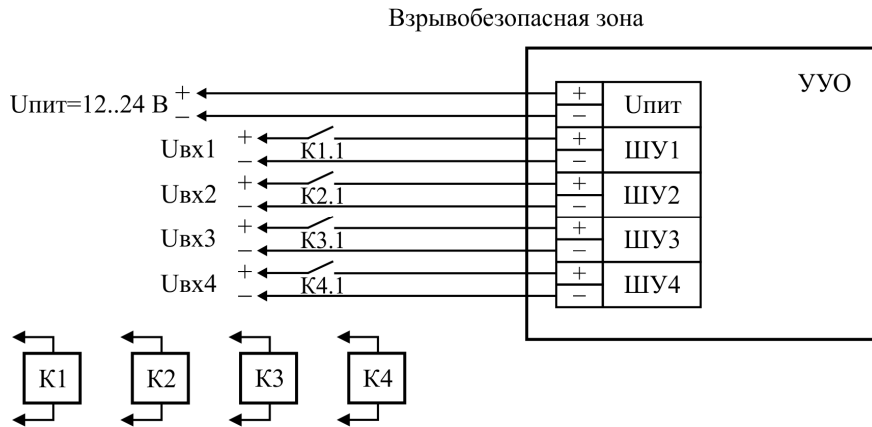
Рисунок 10. Пример схемы подачи внешних управляющих сигналов на УЗО-RGB через транзисторные ключи.
