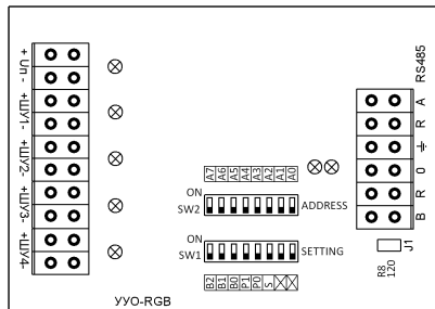
Рисунок 3. Назначение клемм оповещателя ЭКРАН-ИНФО-RGB.
