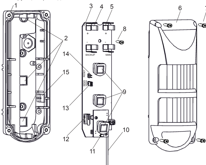
Рисунок 1 – Извещатель
