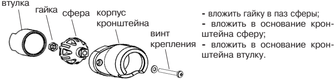
Рисунок 3 – Детали кронштейна
