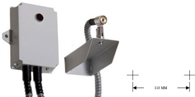
Рис. 1 Спектрон-210, -210-Р и разметка его крепления
