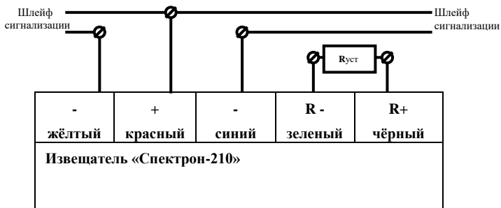
Рис. 2 Схема включения 2-х проводного извещателя
