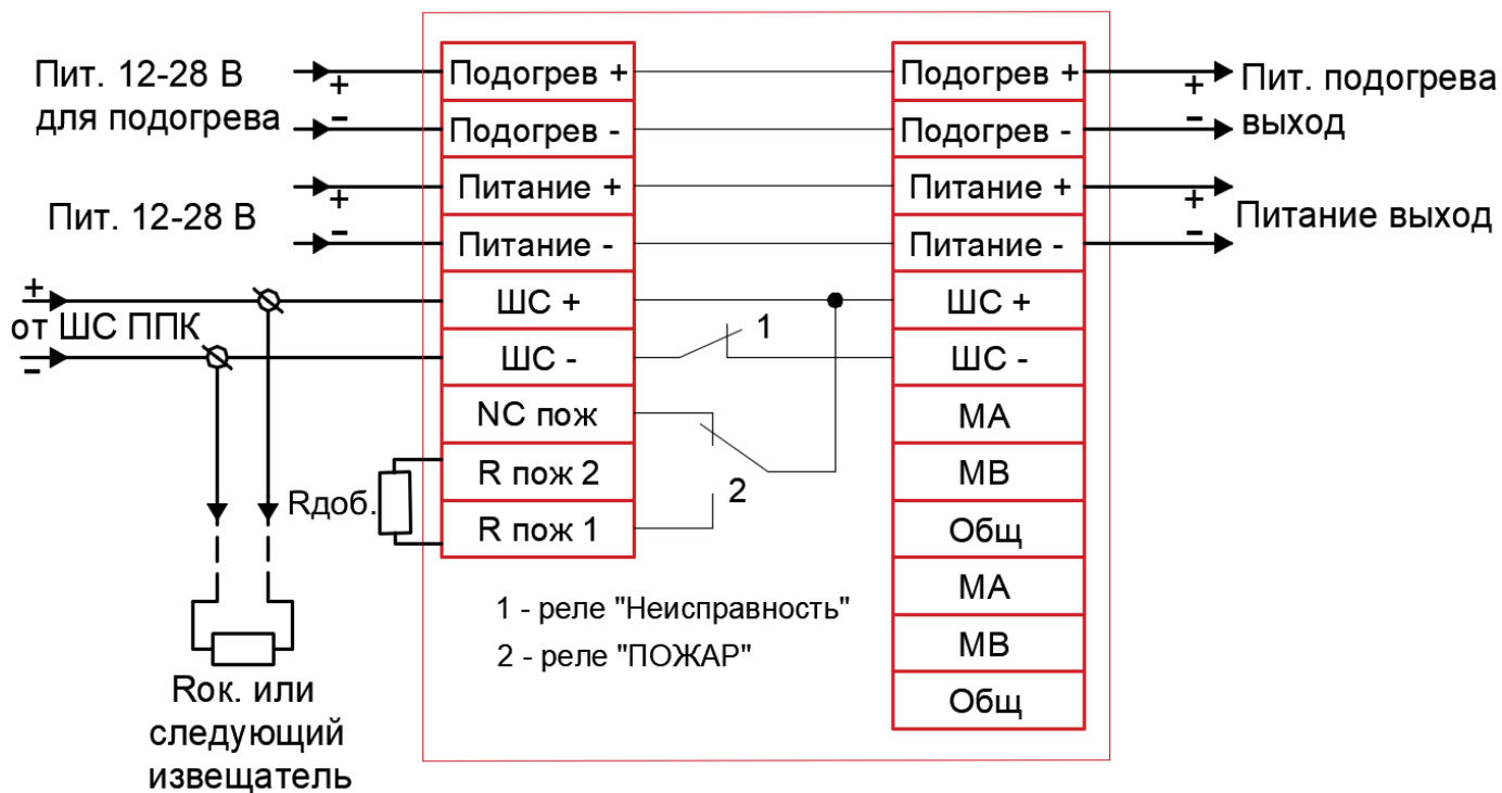
Рисунок 18 – Схема подключения к C2000-AP2 (AP-8) без использования режима «НЕИСПРАВНОСТЬ»
