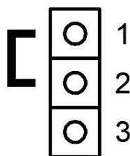
Рисунок 13 – Установка джампера согласующего резистора
